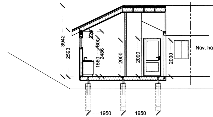
Snið B-B
