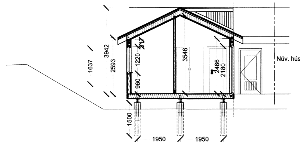
Snið A-A
