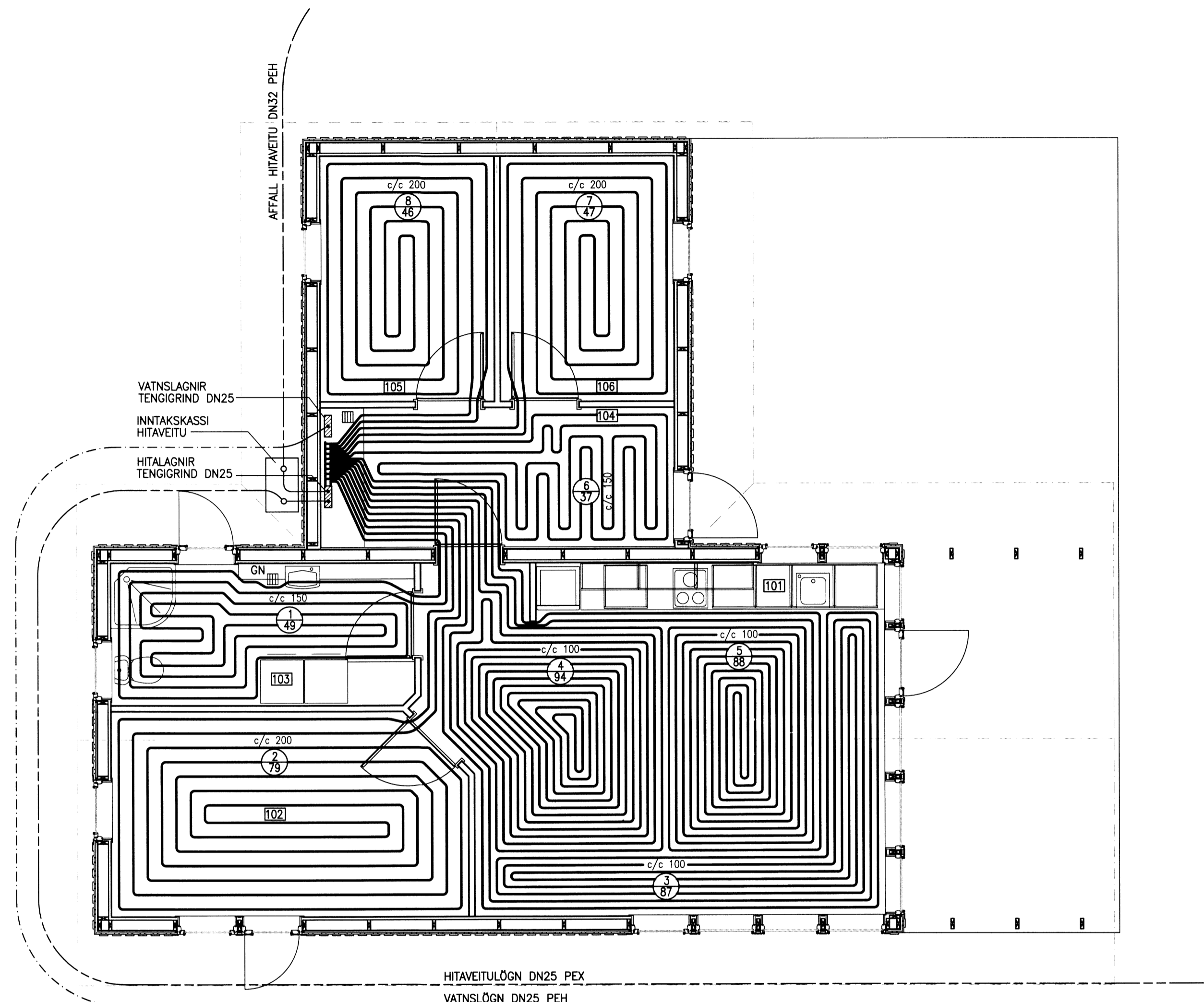
GRUNNMYND HITALAGNIR 1:50
