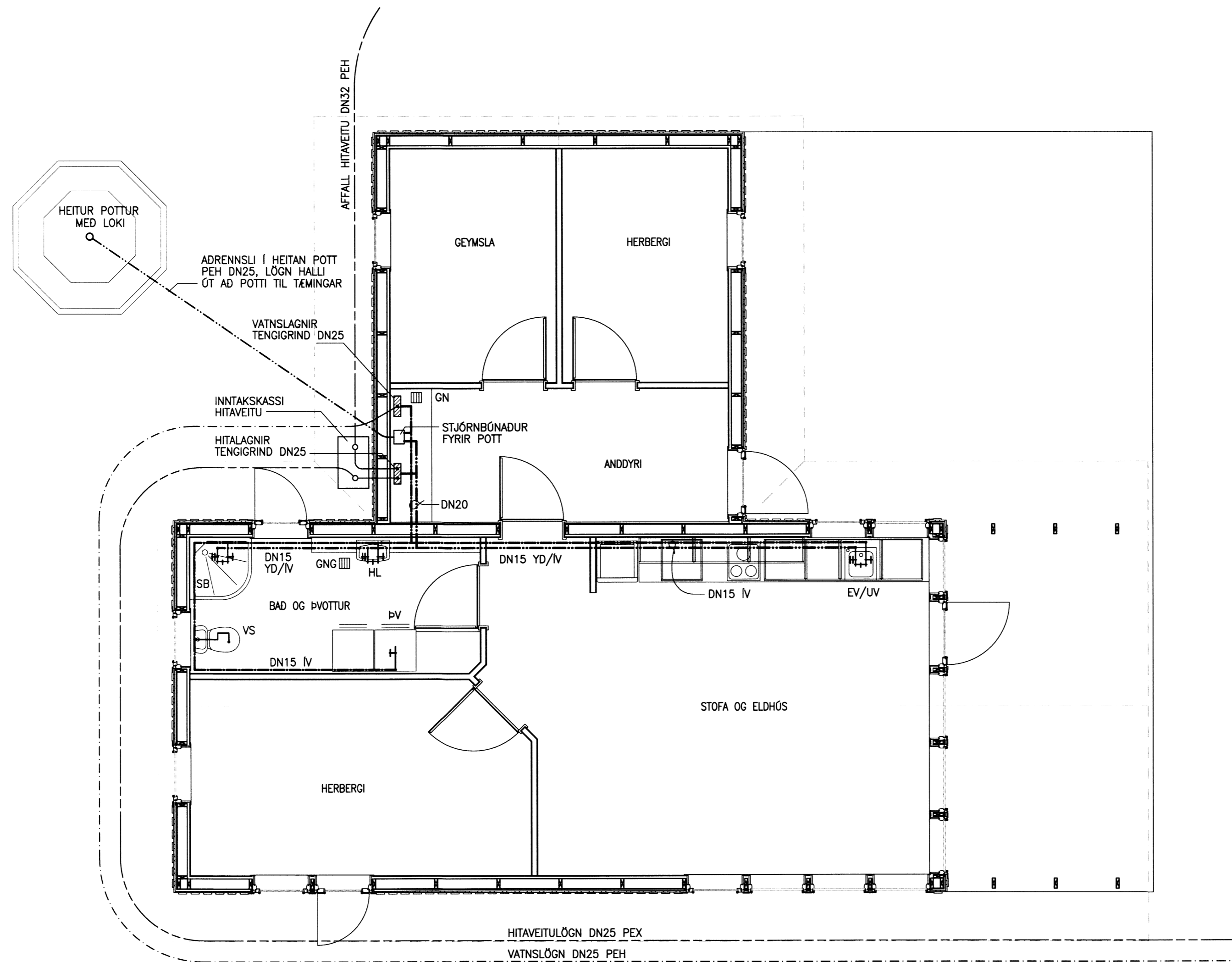
GRUNNMYND VATNSLAGNIR 1:50
