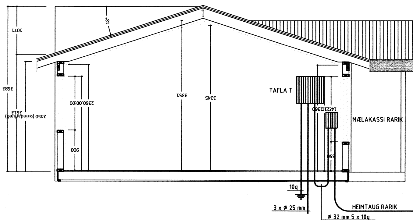
SNID A-A
