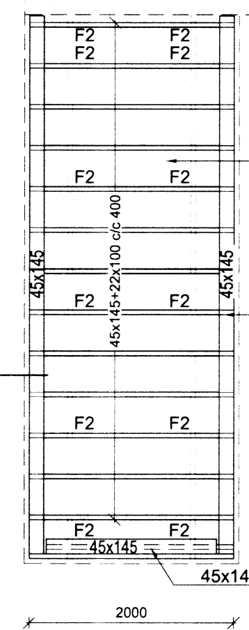
Grunnmynd gólfs M 1:50
