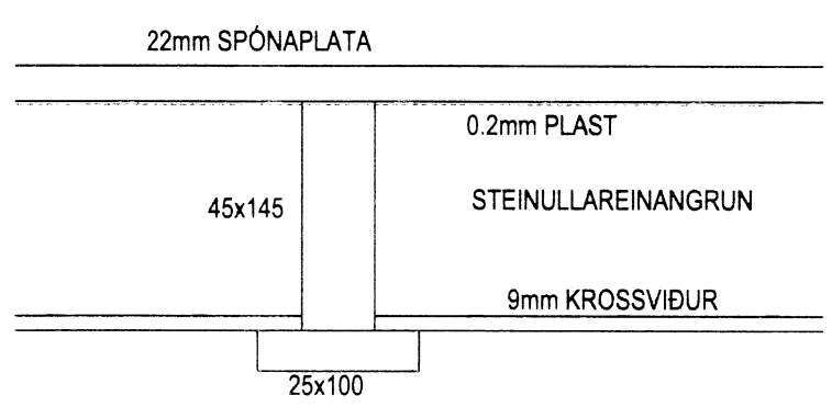
Uppbygging gólfs M 1:5
