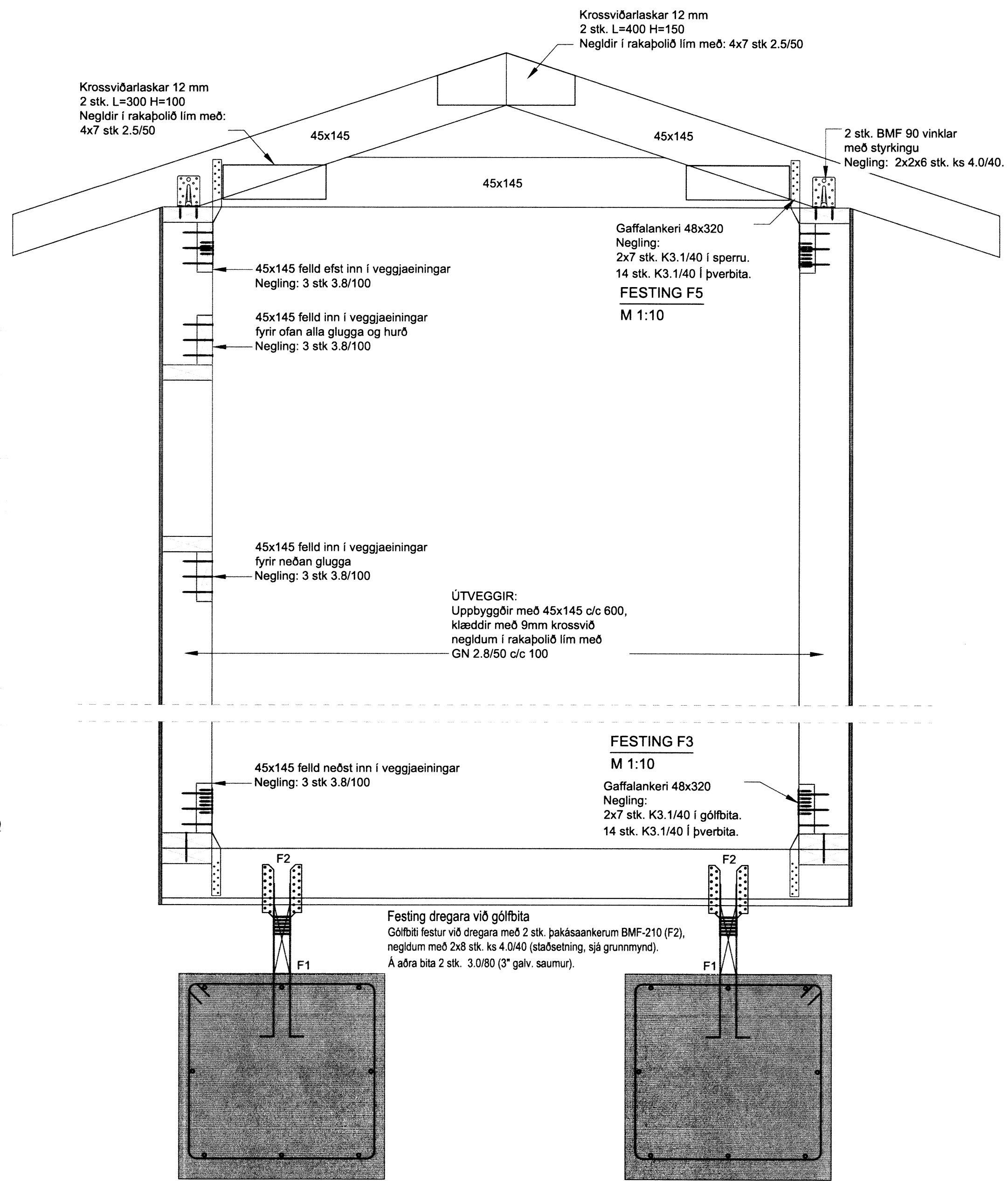
AA Snið M 1:10
