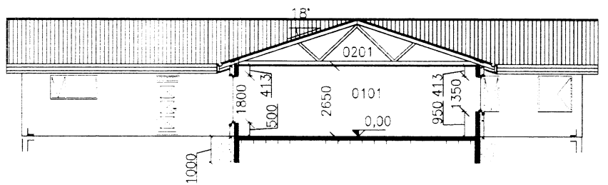
A SNIB 001 1:100
