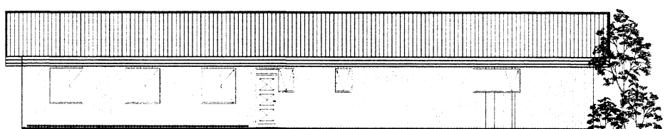
ÚTLIT NORÐUR 1:100
