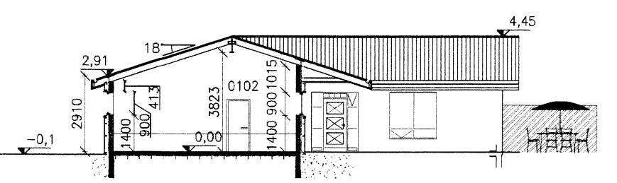
B SNIB 001 1:100
