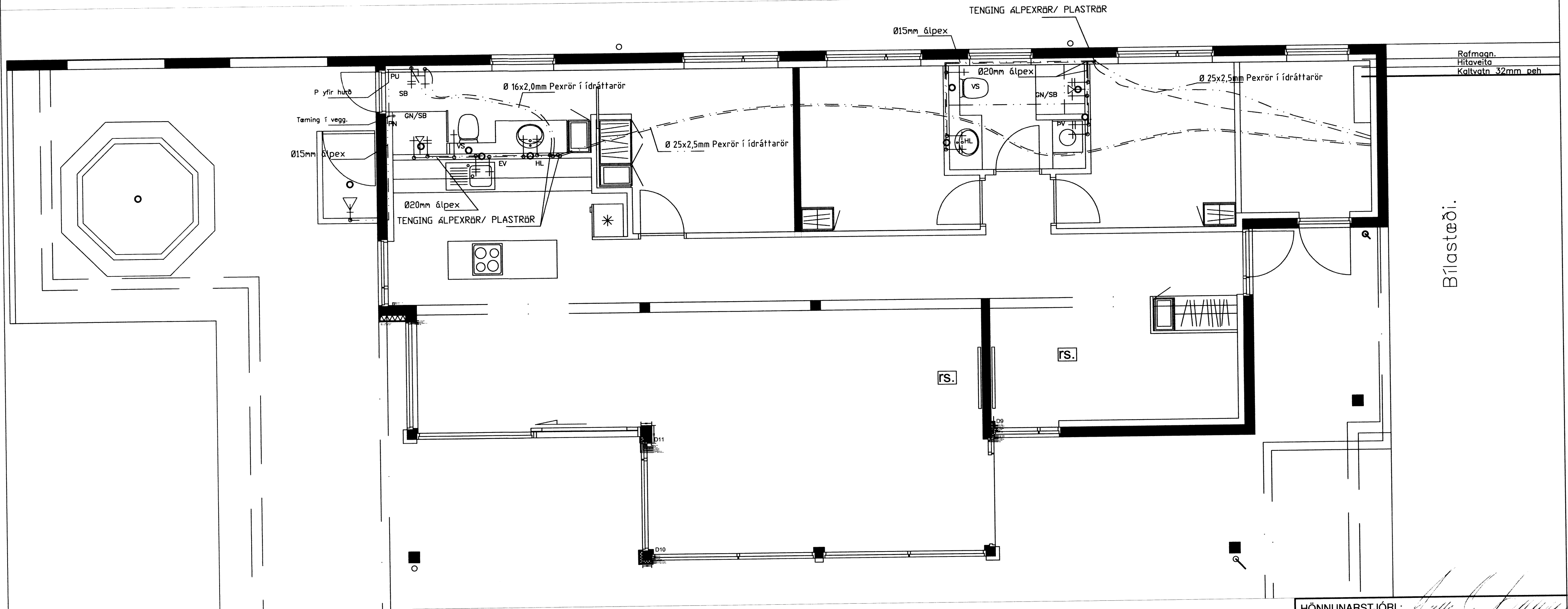
Grunnmynd Mkv. 1:50
