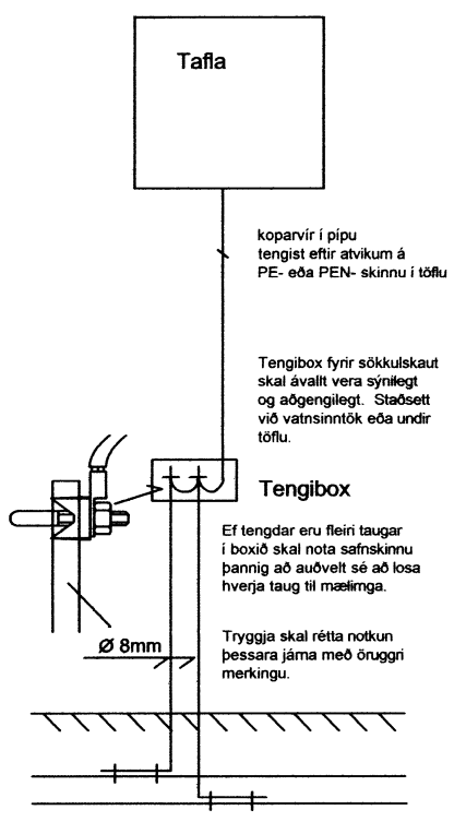
Snið í töfluvegg
