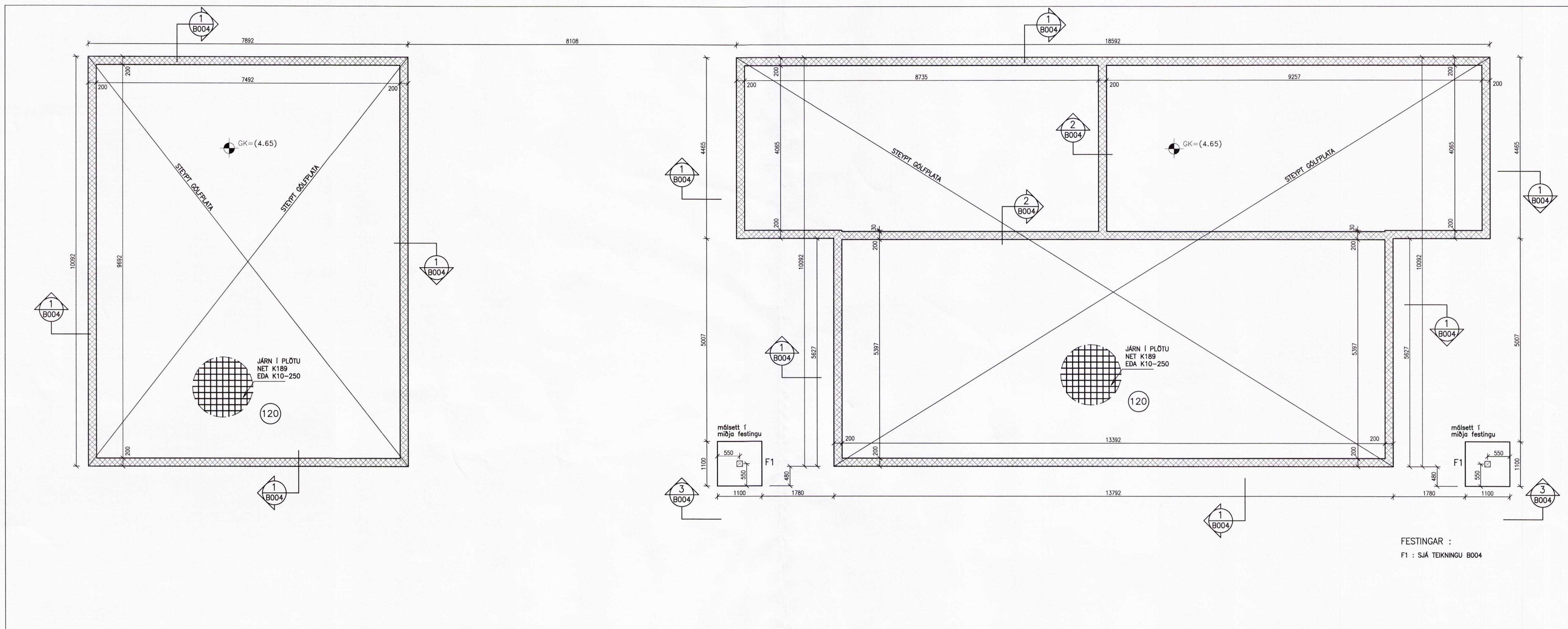
GRUNNMYND UNDIRSTÖÐUR GESTAHÚS 1:50
