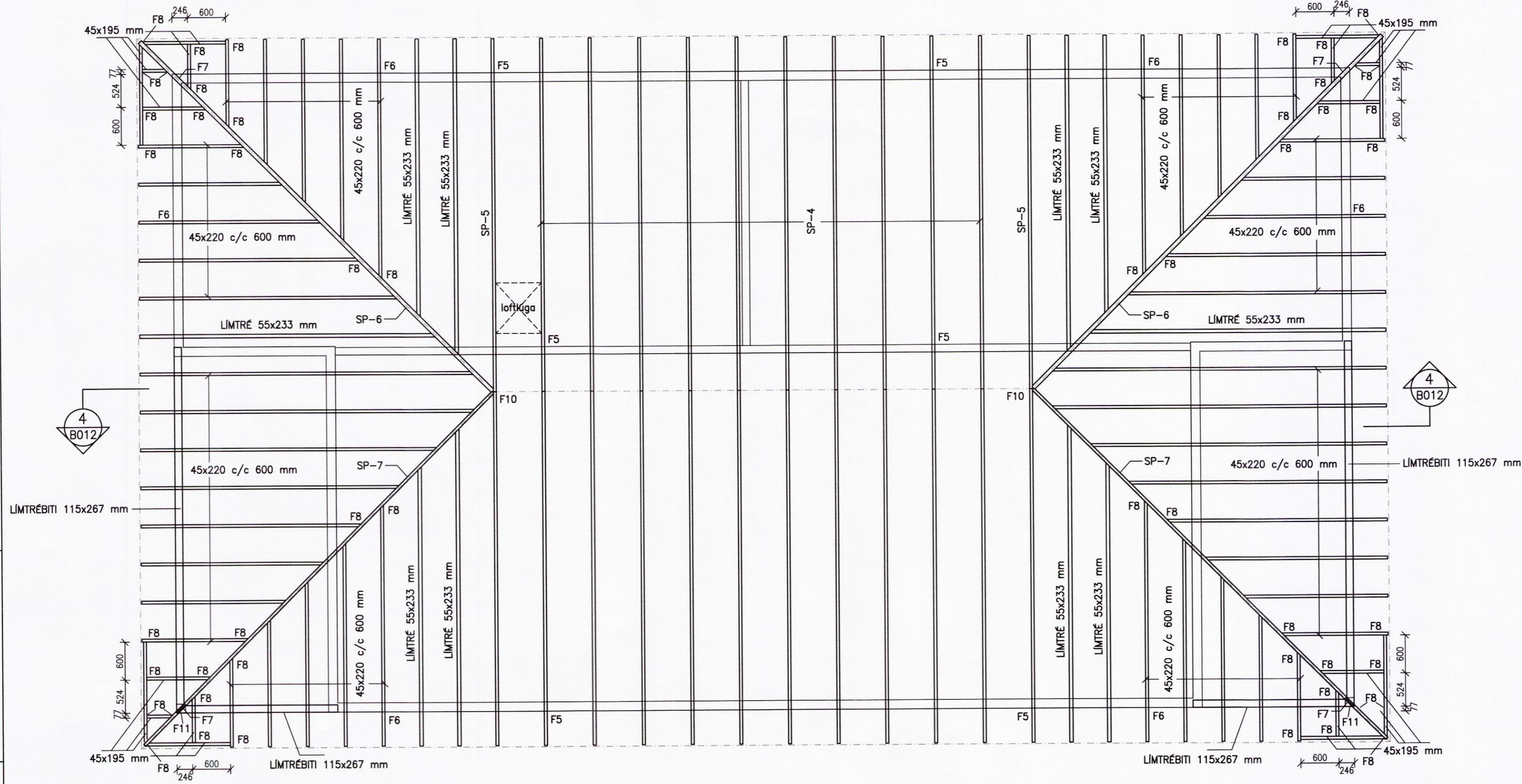
SPERRUPLAN IBÚÐARHÚS 1:50
