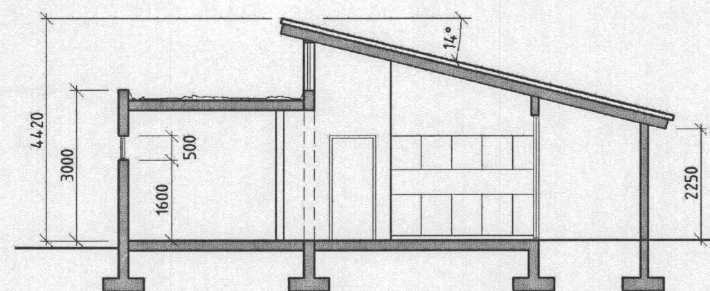
Sníð A-A 1:100
