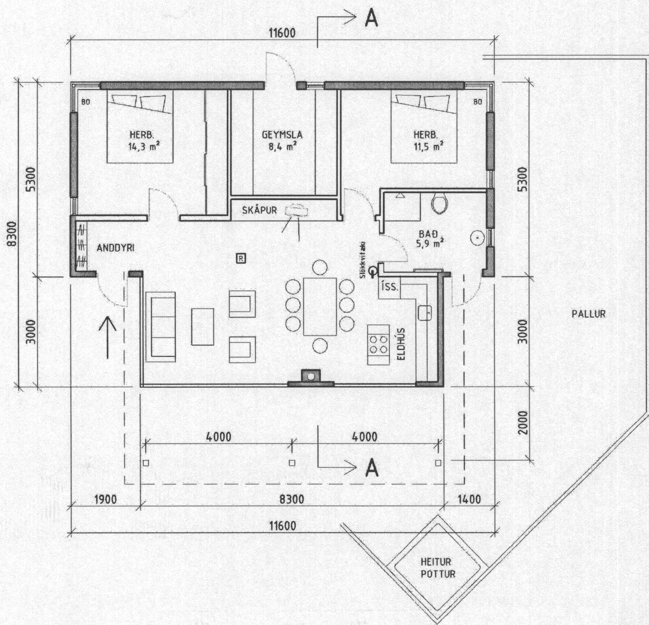
Grunnmynd 86,4 m 2 1:100
