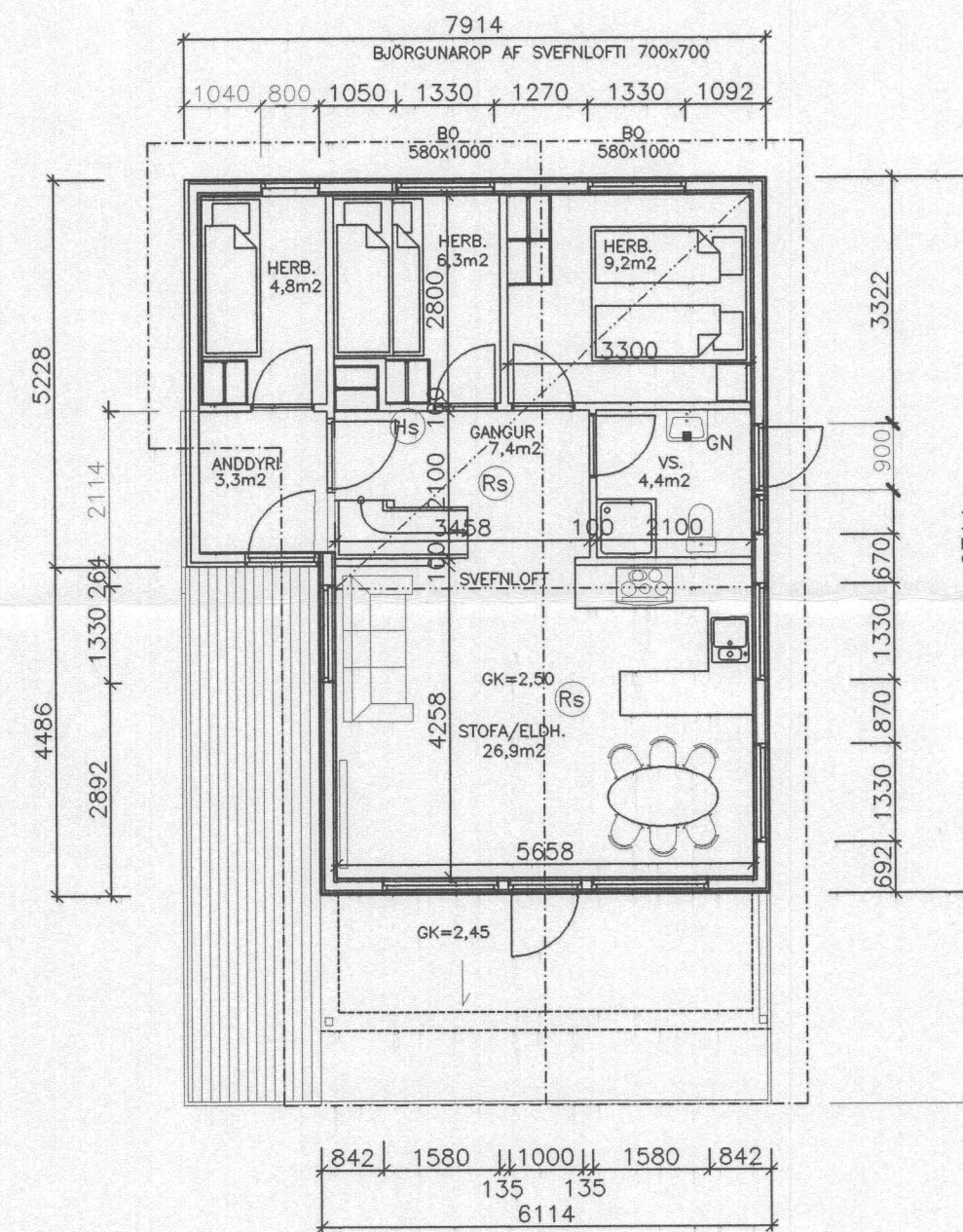
GRUNNMYND MATSHL. 01
