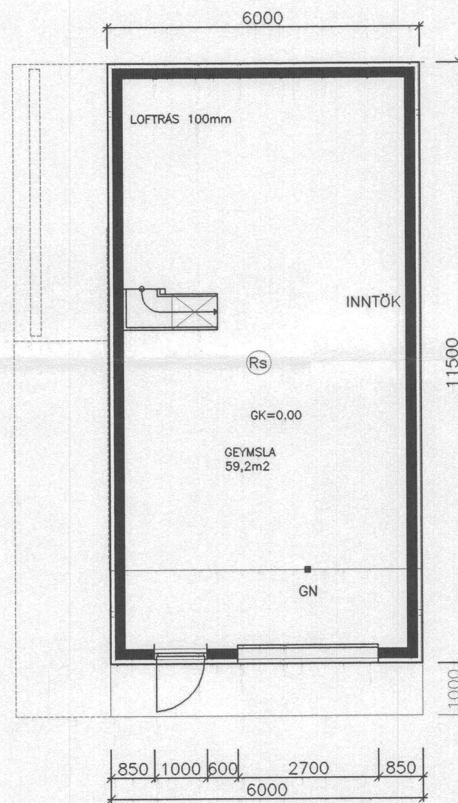
GRUNNMYND KJALLARA
