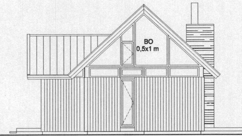
austur m 1:100
