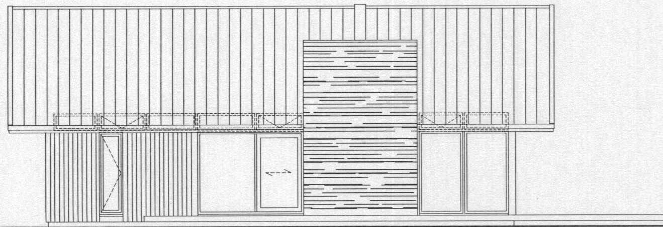
norður með efri gluggum m 1:100
