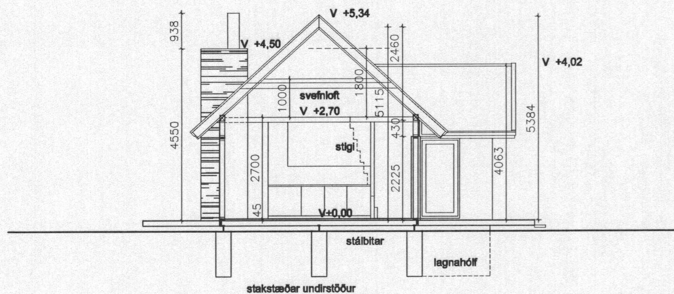
snið AA m 1:100
