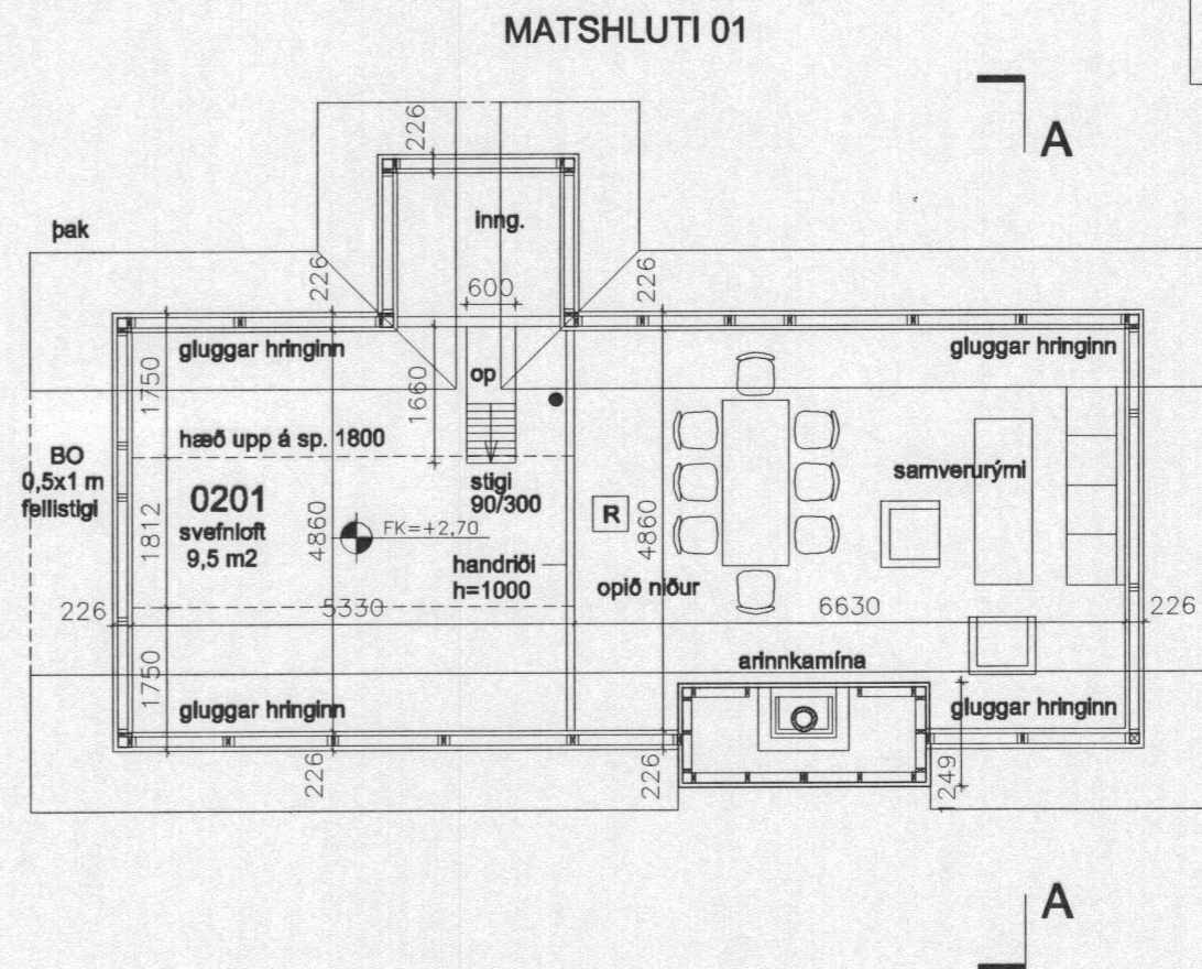
grunnmynd svefnloft m 1:100
