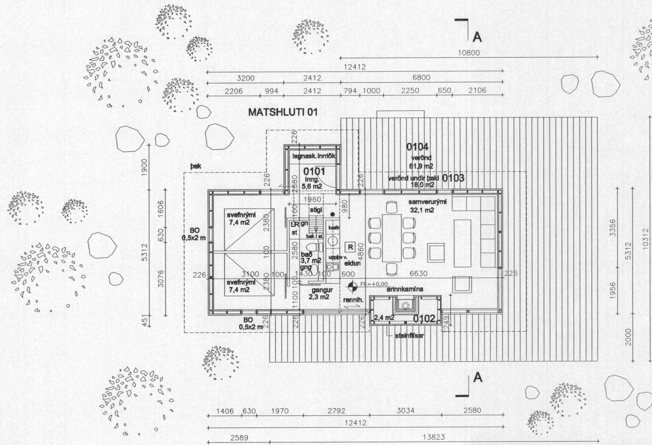
grunnmynd jarðhæð m 1:100
