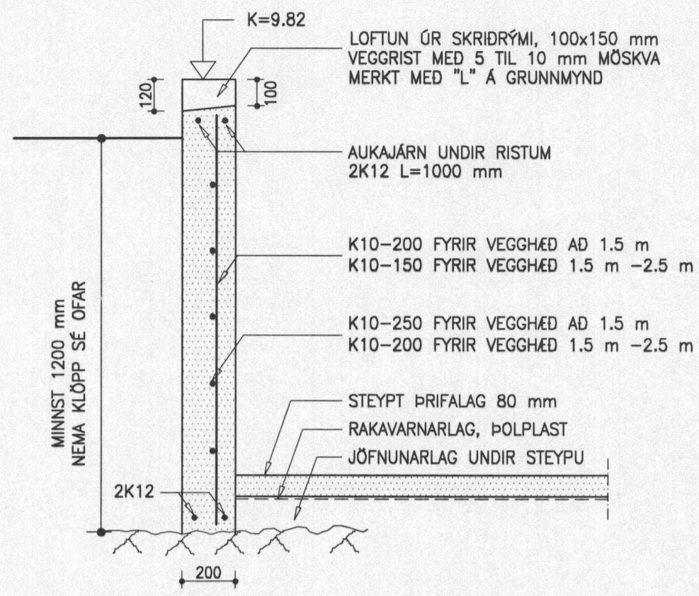
SNID 1-1 1:20
