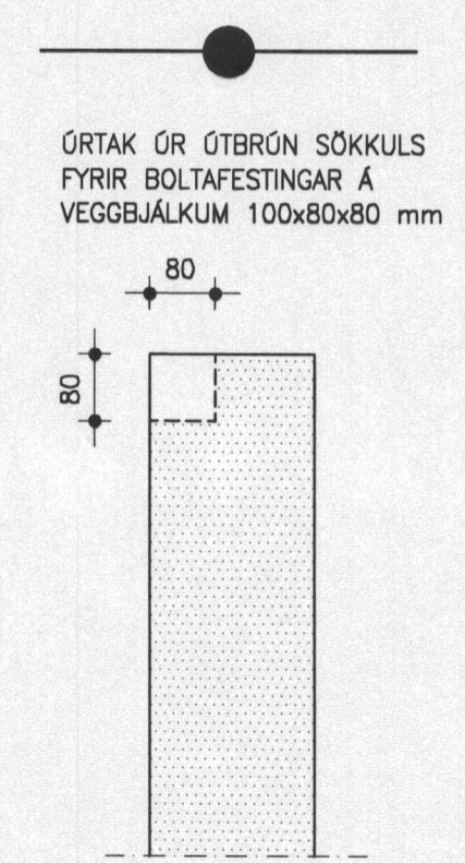
BOLTAÚRTAK 1:10
