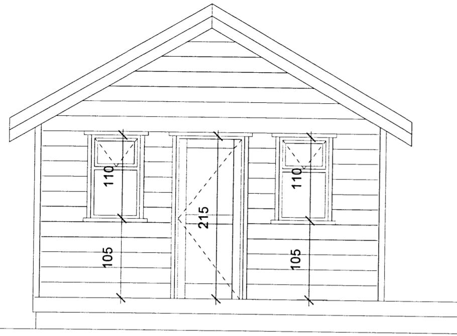
Útlit suðvestur, m.kv.: 1:50
