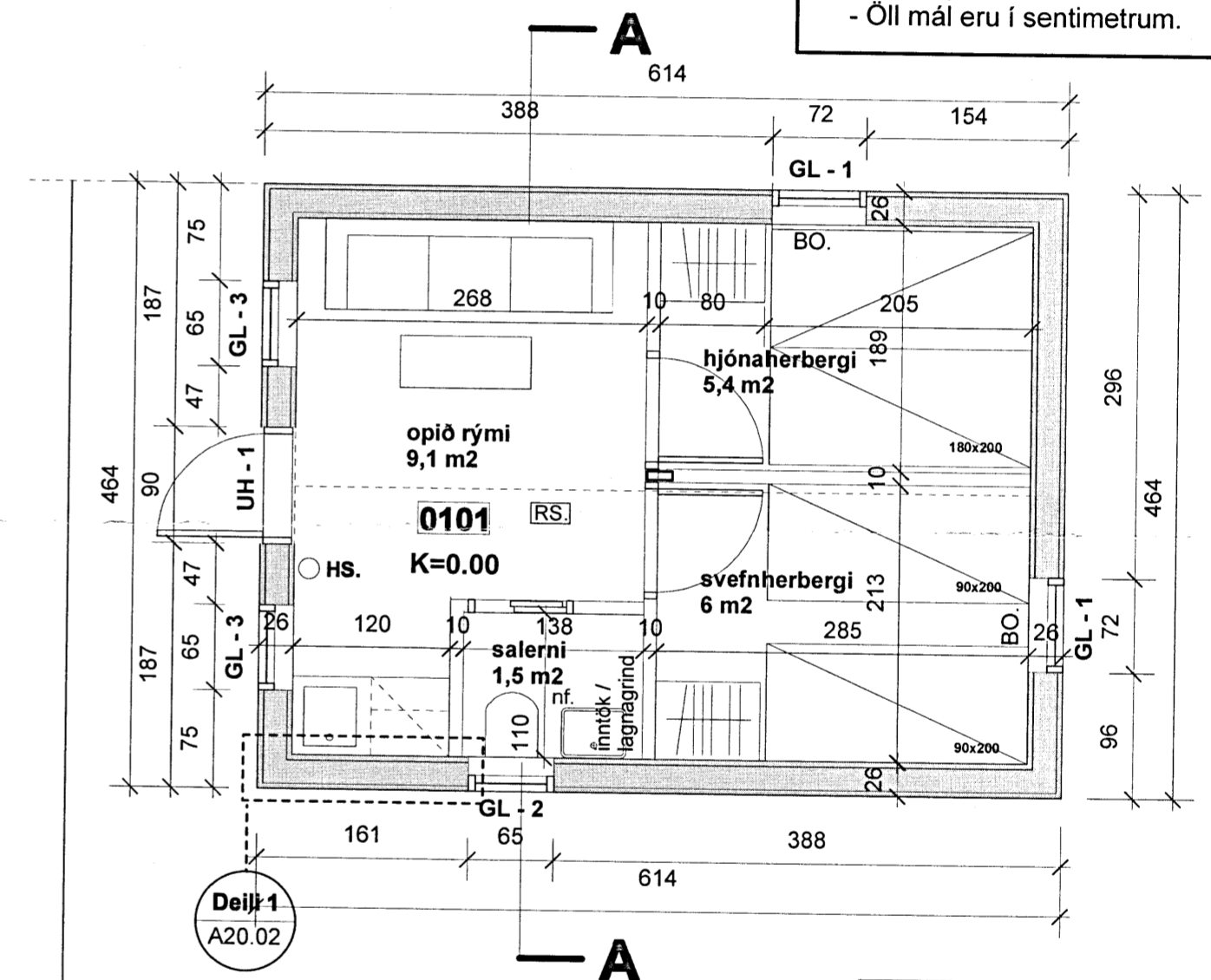
Grunnmynd, m.kv.: 1:50
