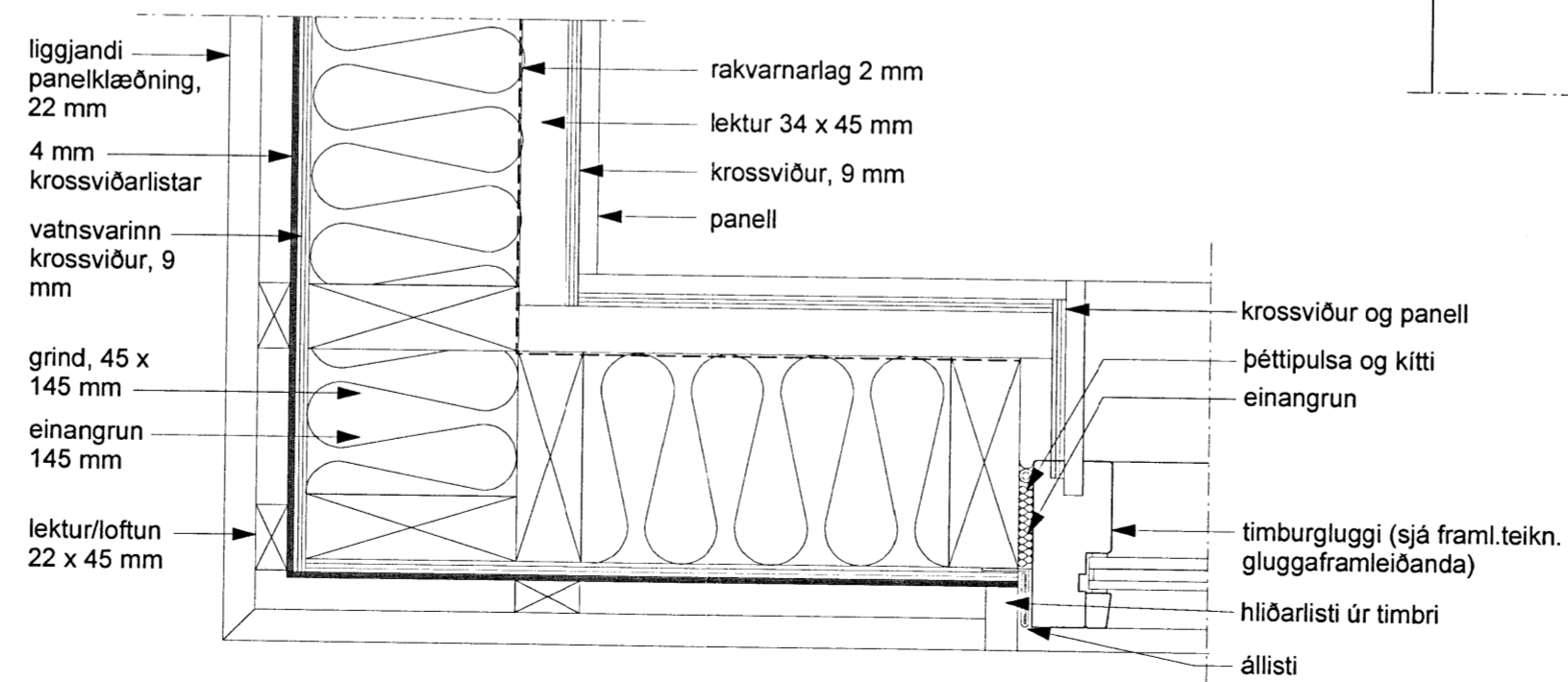
Deili 1: Lárétt deili við horn og glugga, m.kv.: 1:5
