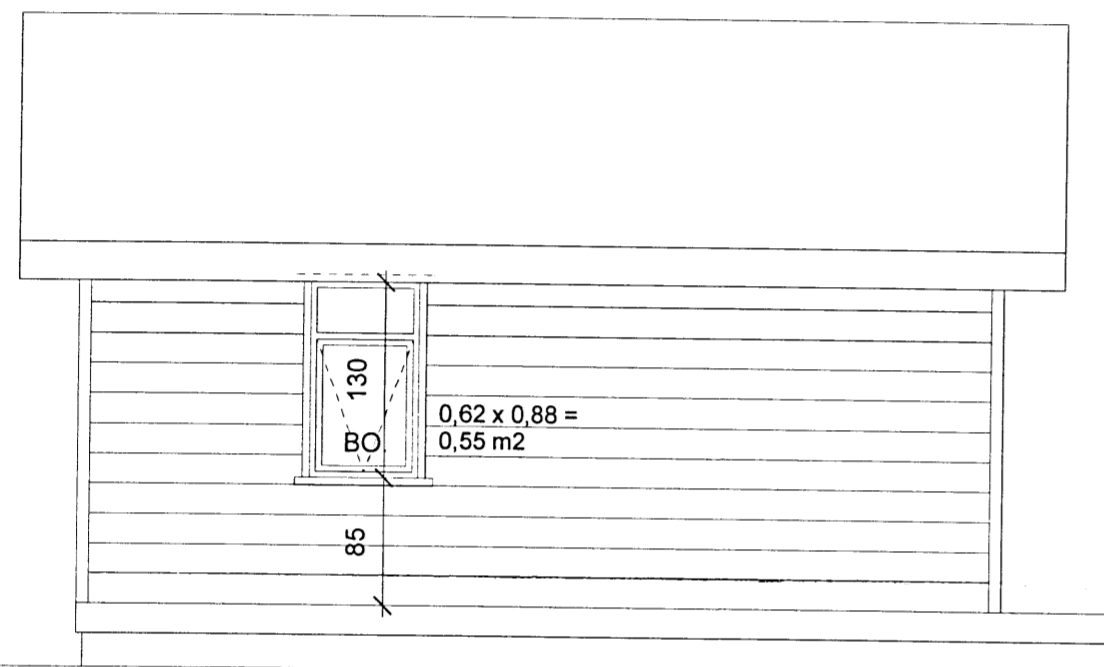
Útlit norðvestur, m.kv.: 1:50
