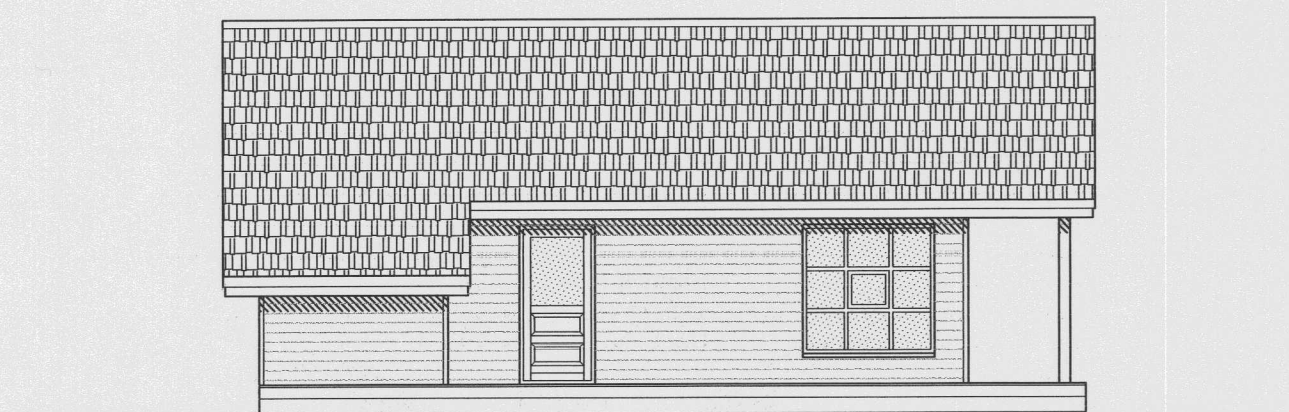
ÚTLIT VESTUR
