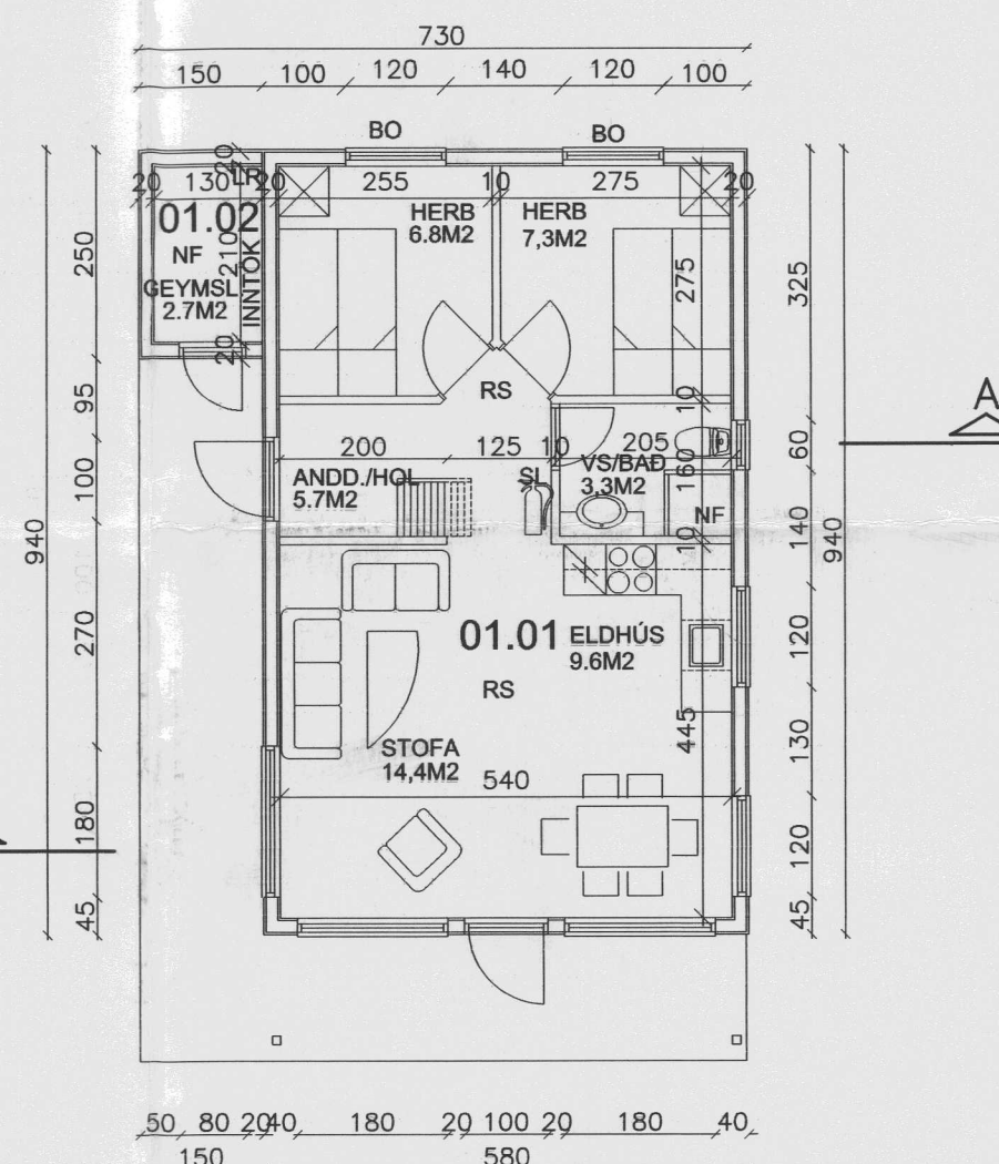
GRUNNMYND
