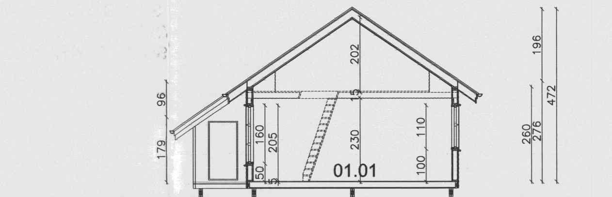
SKURÐUR A.
