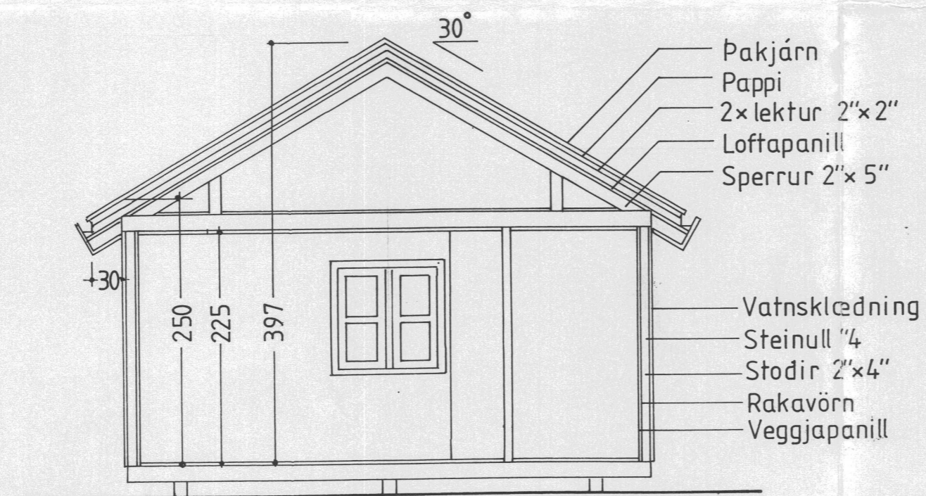
SNEIÐING A-A
