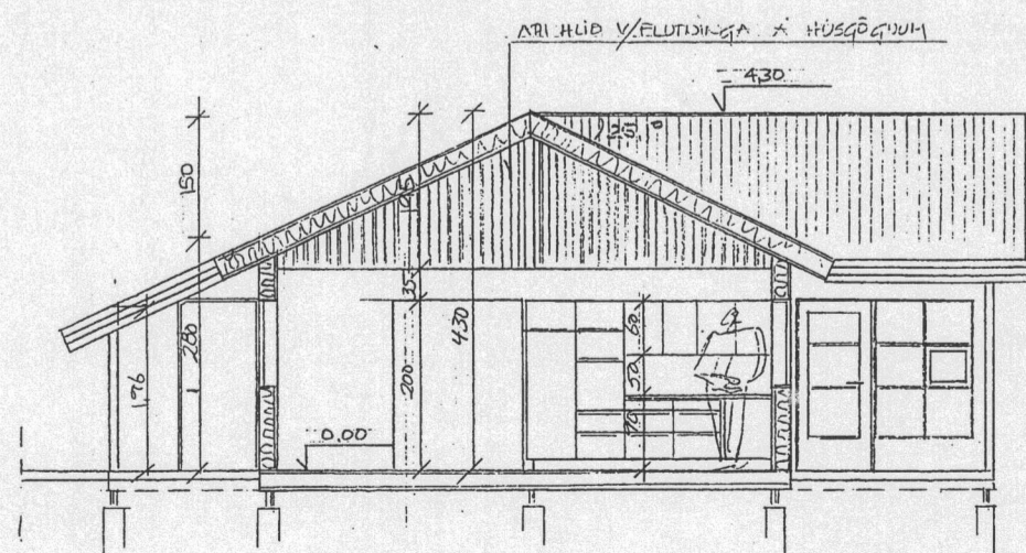
Snið A-A 1:100
