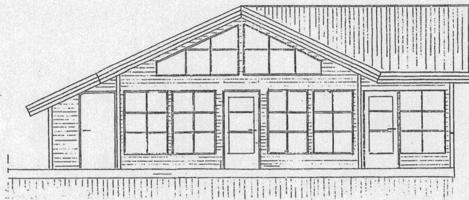
Vesturhlið 1:100
