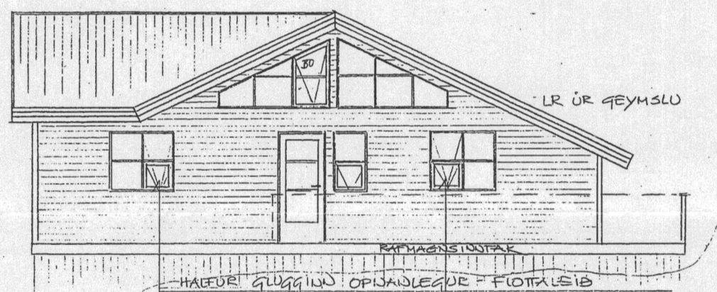
Austurhlið 1:100
