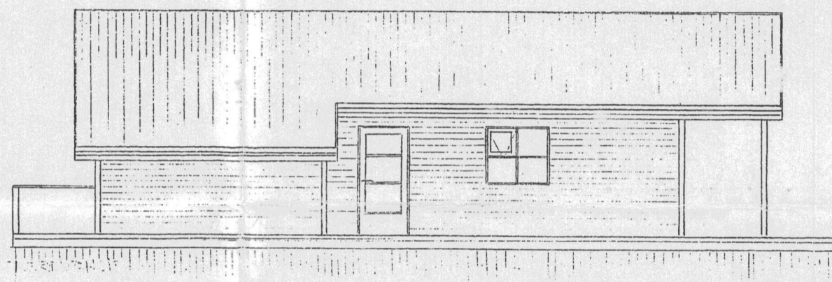
Norðurhlið 1:100
