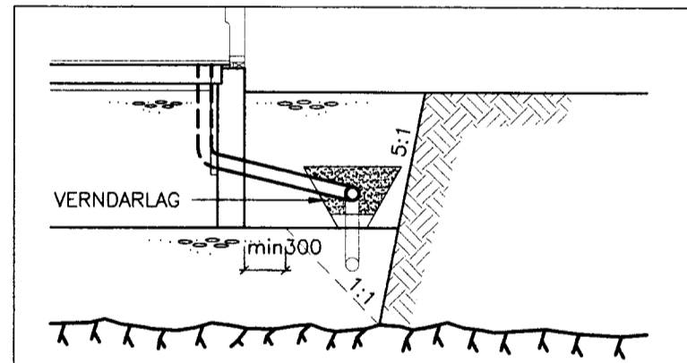
SNID VID SÖKKUL Mkv. 1:50
