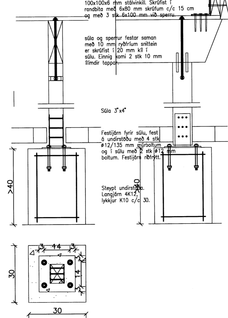
1.5 Sérmynd 1.5. 1:10.
