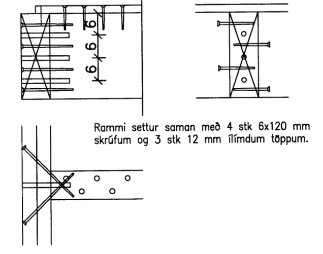
1.7 Sérmynd 1.7. 1:10.
