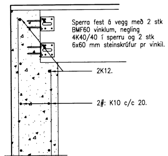
1.2 Sérmynd 1.2. 1:10.
