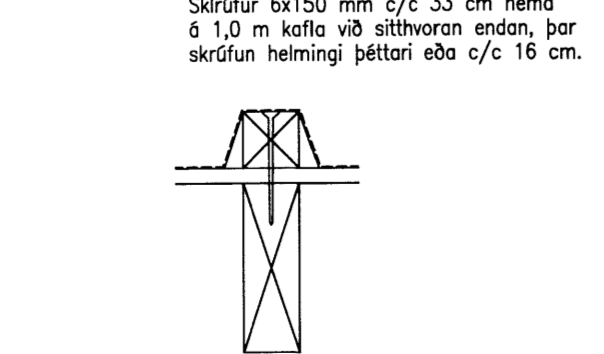
1.7 Sérmynd 1.7. 1:10.
