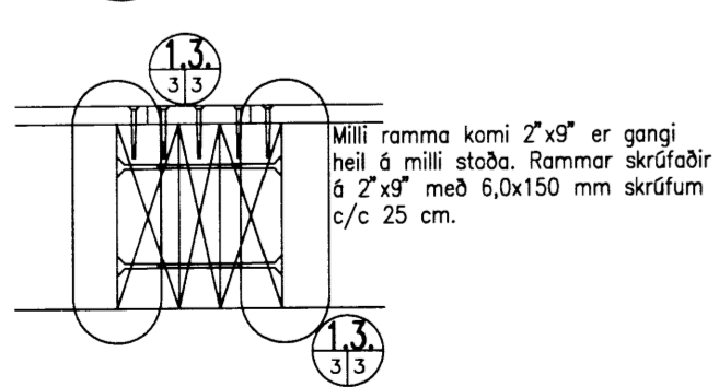
1.2 Sérmynd 1.2. 1:10.
