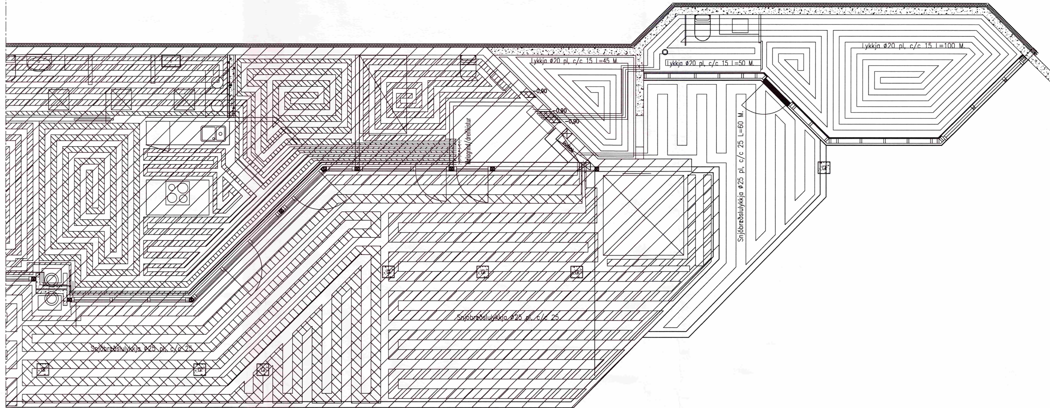
Hitalögn: Rúmmynd. 1:50.
