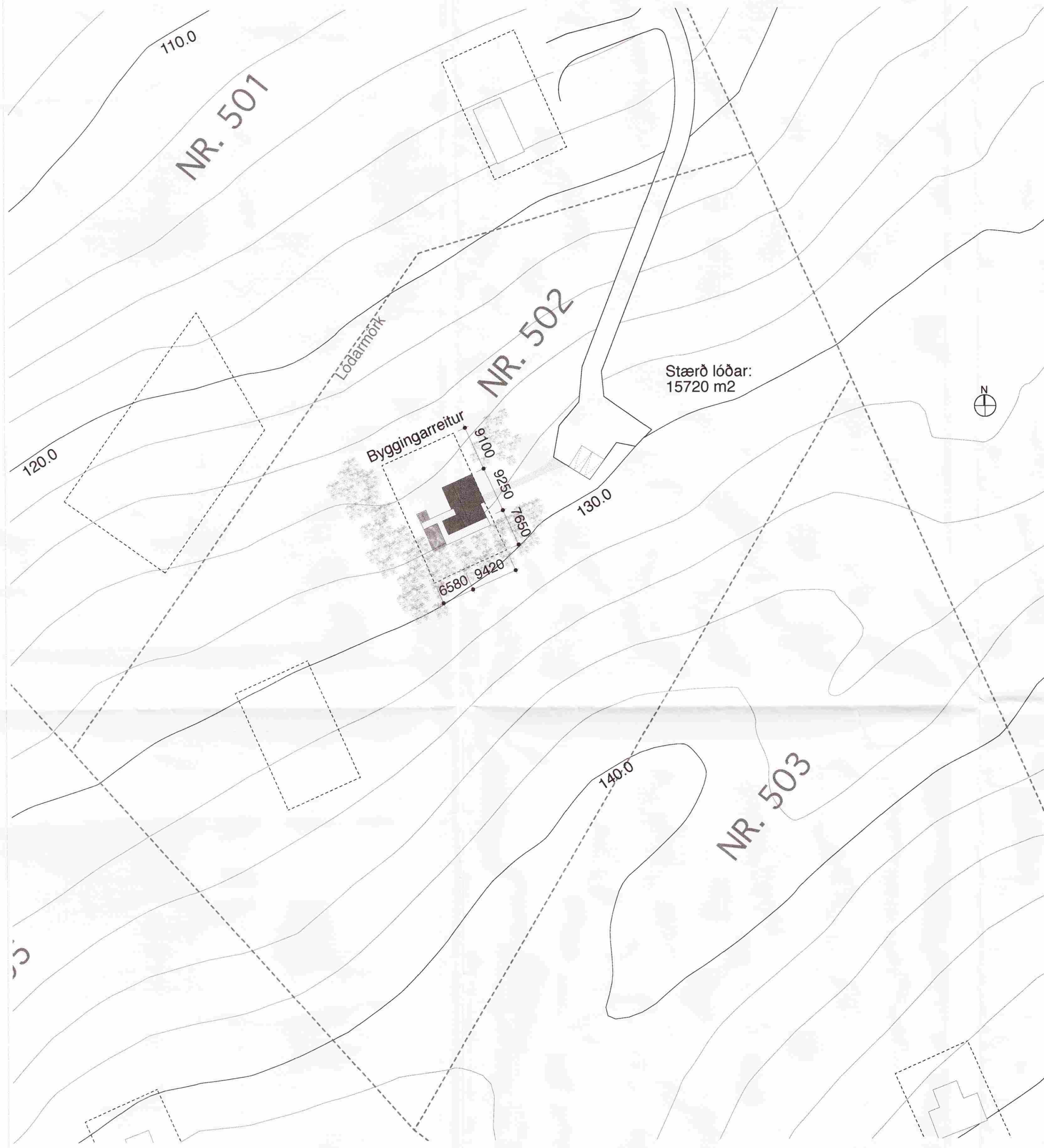
AFSTÖÐUMYND MKV. 1:500
