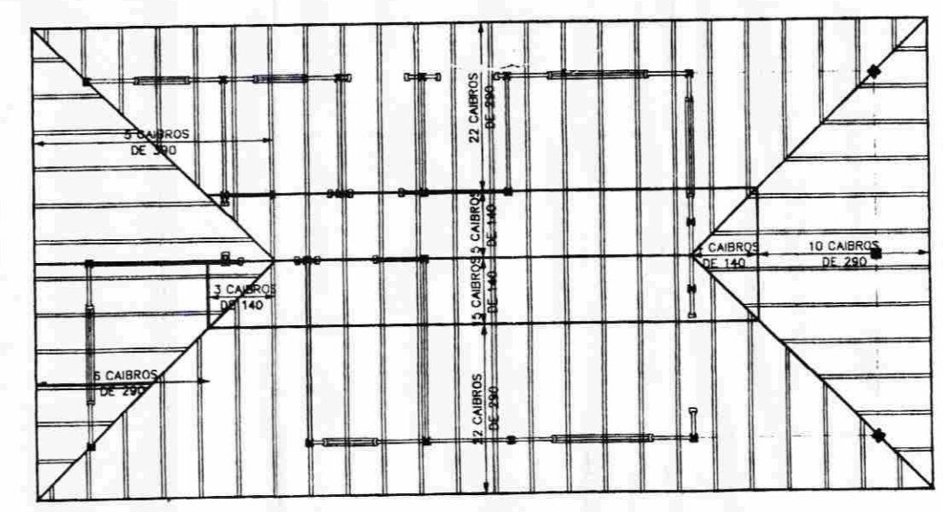
PLANTA DE CAIBROS ESCALA 1:100
