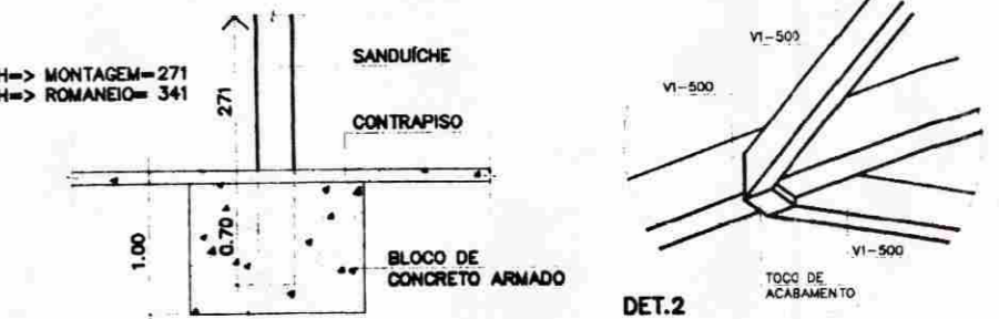
DET.2 DETALHE DA FIXAÇÃO DOS PILARES MONTADOS SANDUICHE
