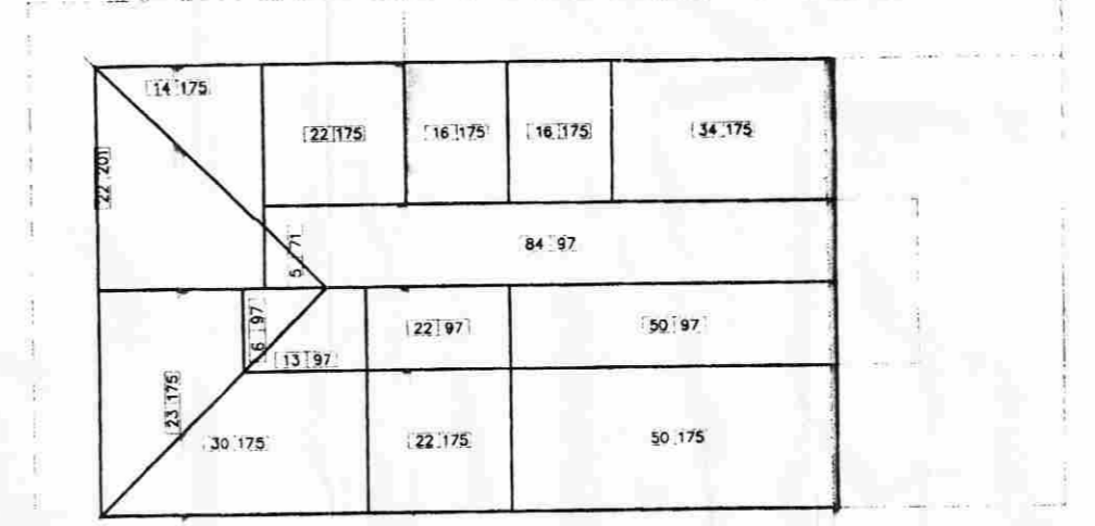
PLANTA DO FORRO *MEDIDAS DE EIXO NO PLANO HORIZONTAL ESCALA 1:100
