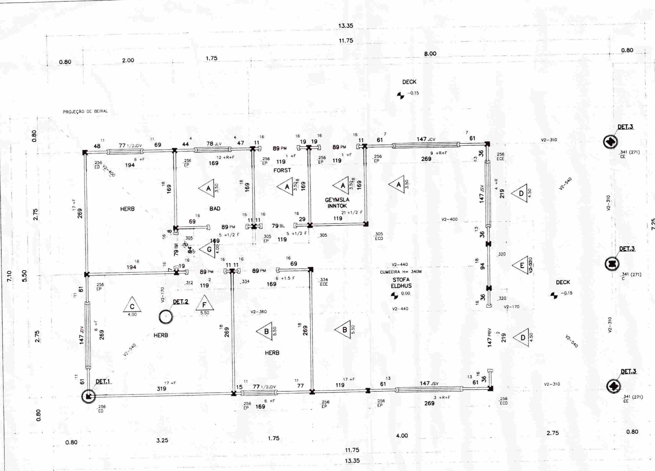
PLANTA DO FORRO *MEDIDAS DE EIXO NO PLANO HORIZONTAL ESCALA 1:100
