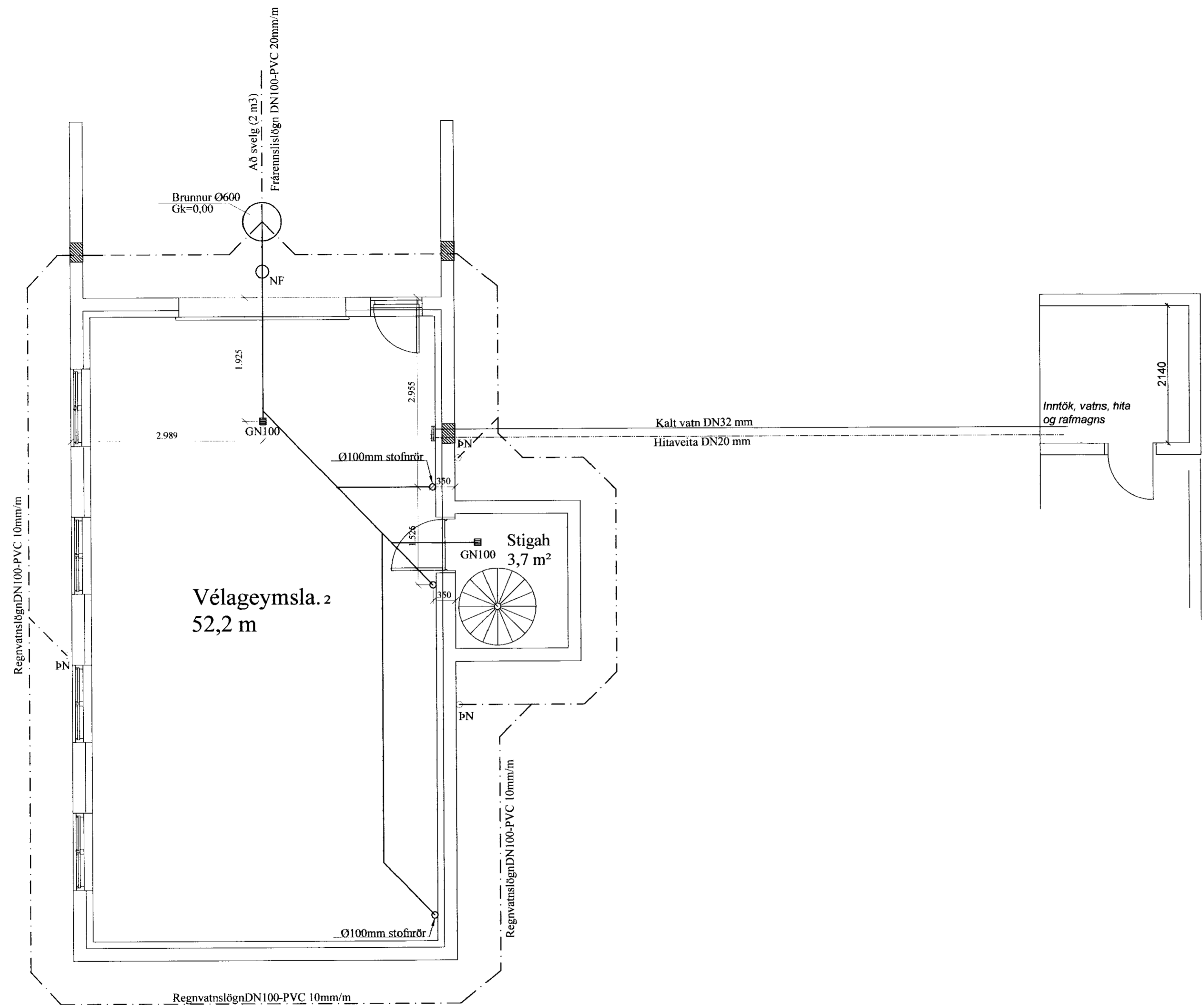
Grunnmynd
