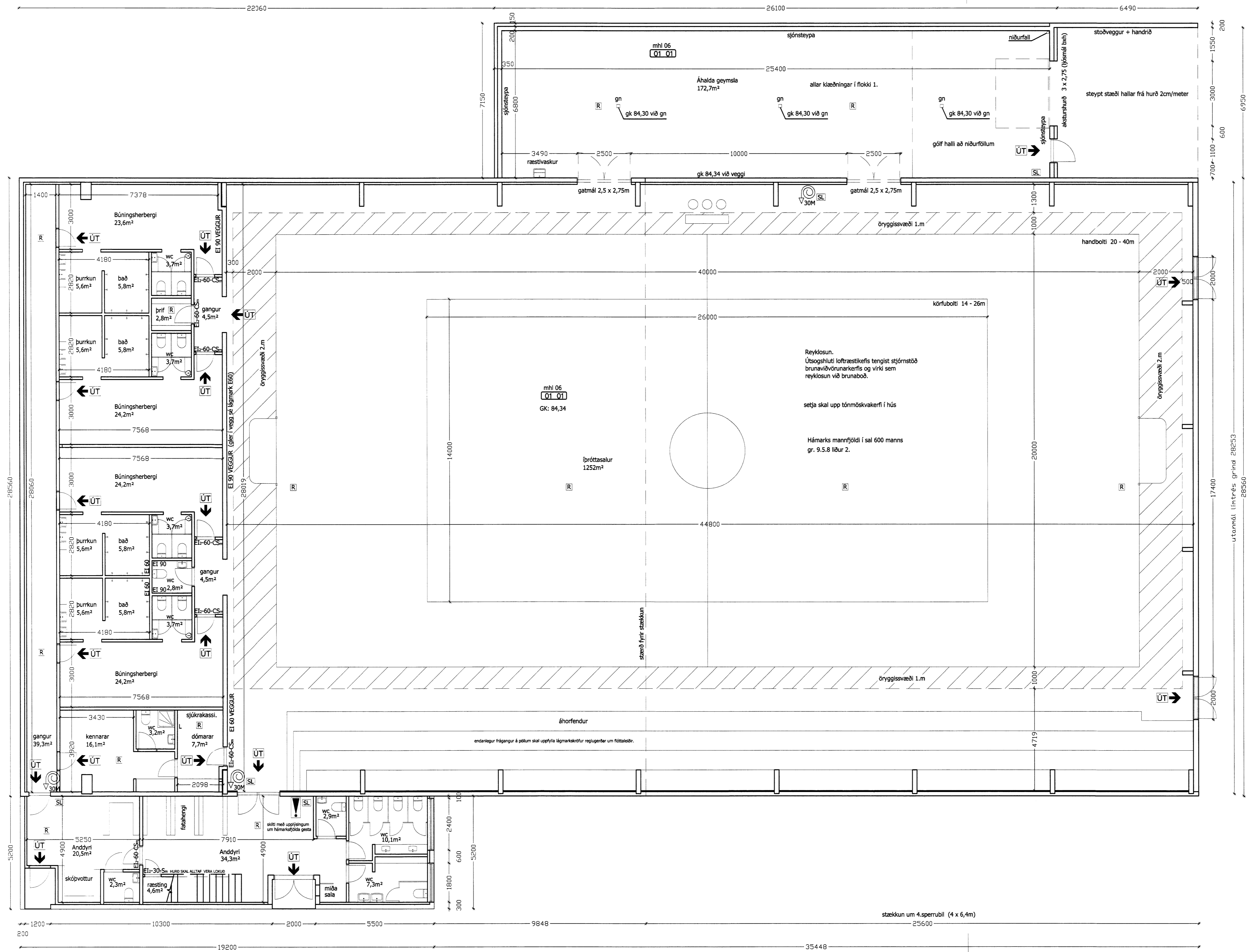
GRUNNMÝND 1. HÆÐ 1:100
