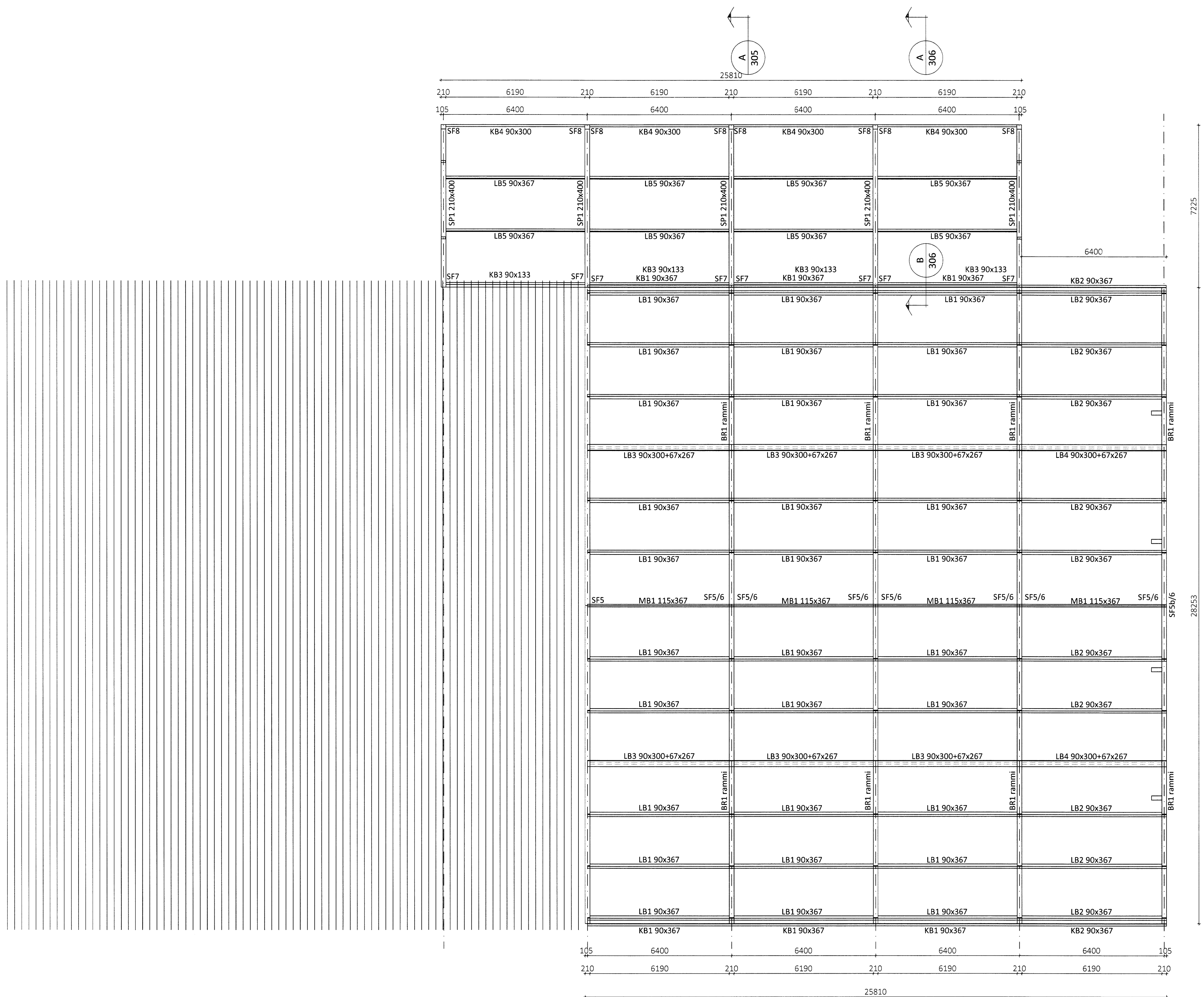
ÞAKMYND Mkv. 1:100
