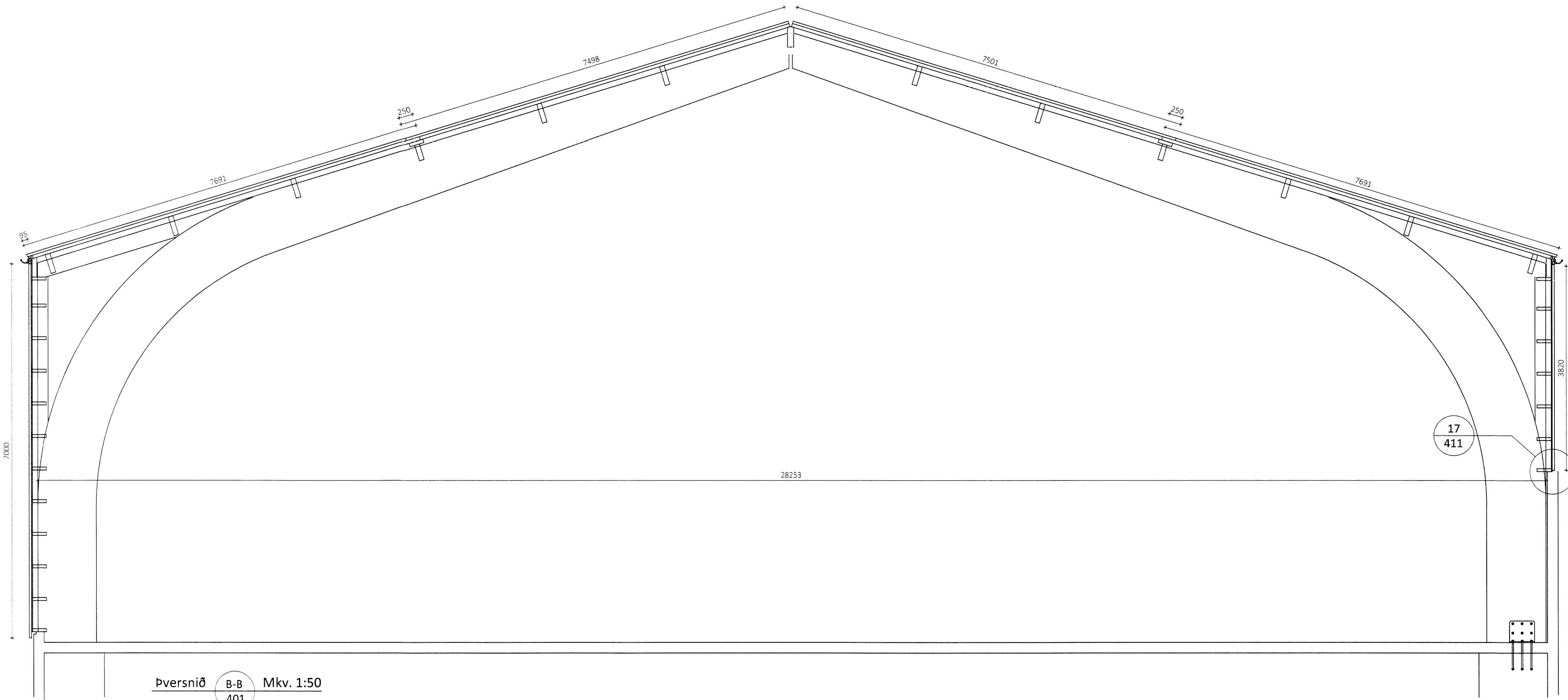
Þversnið A-A Mkv. 1:50 401
