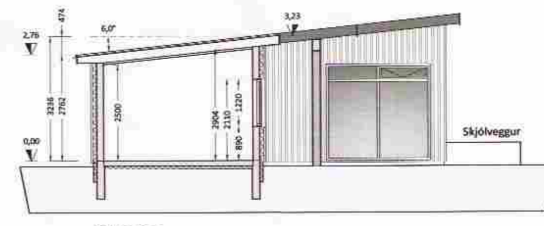
SNID C-C Mkv. 1:100
