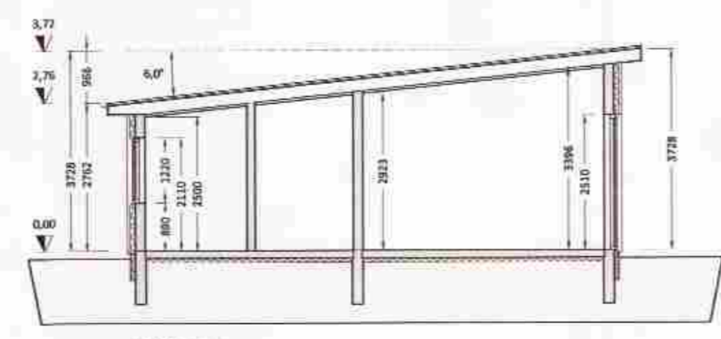
SNID B-B Mkv. 1:100
