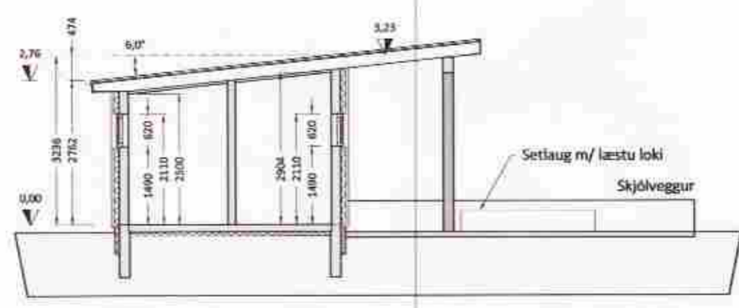
SNID A-A Mkv. 1:100
