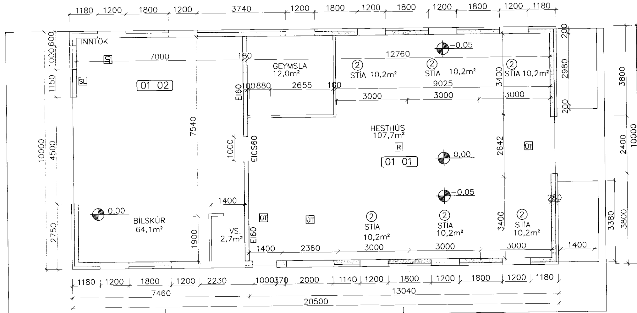
GRUNNMYND 1:100
