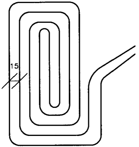
Dæmigerð gólfhitaslaufa
