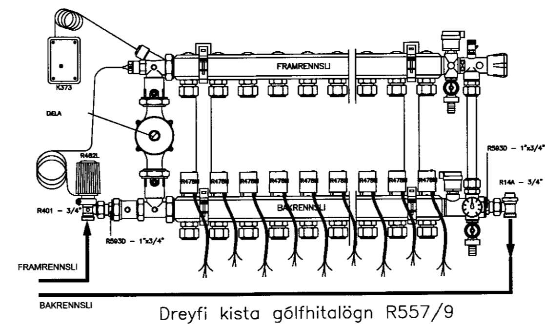
( SKEMATÍSK MYND )
