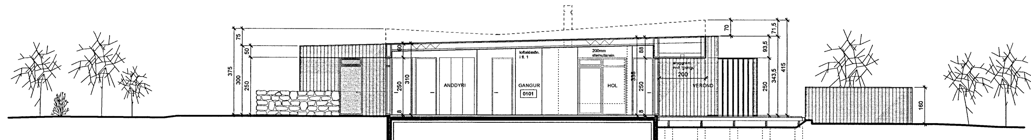
SNÍÐ / ÚTLIT B B
