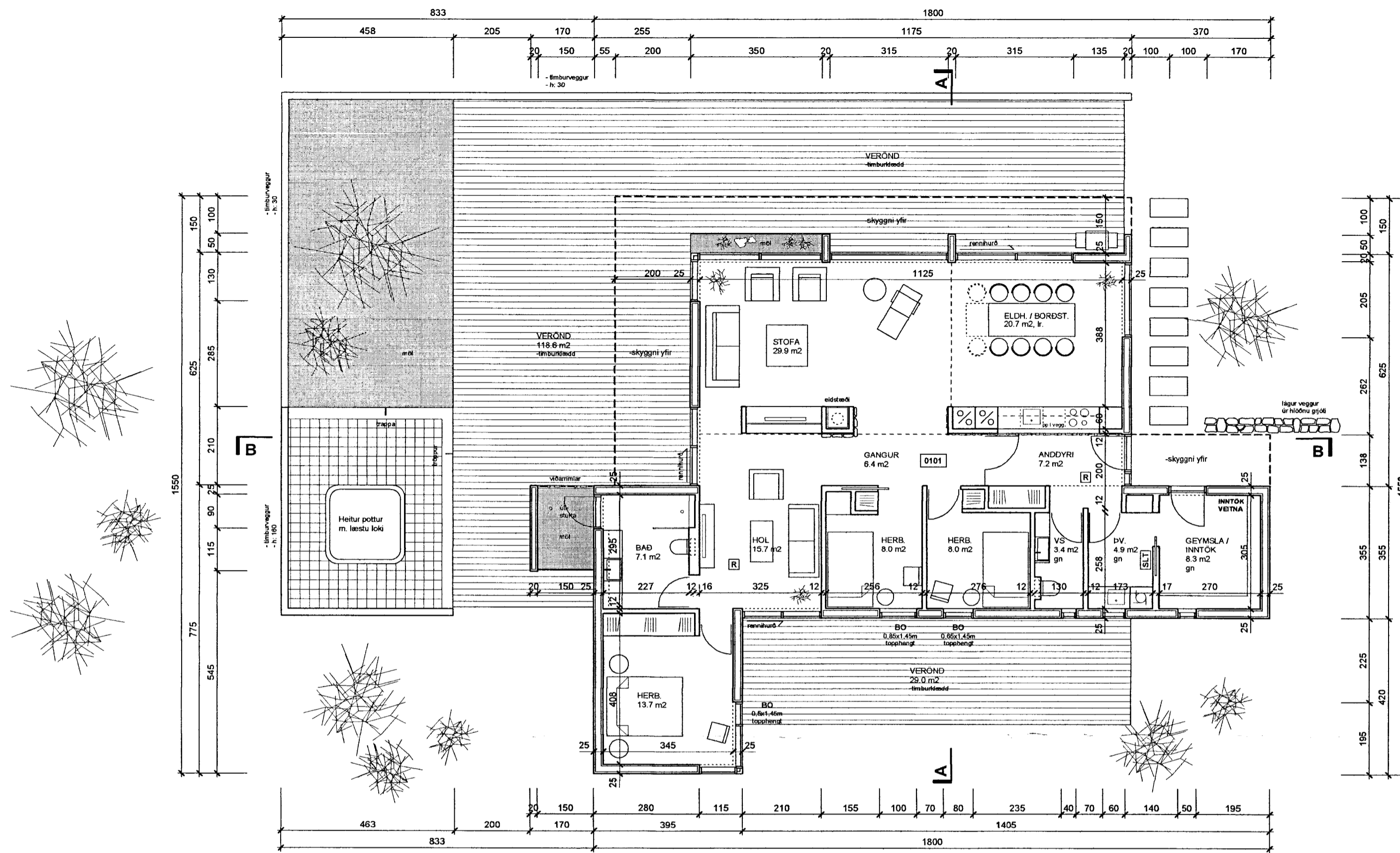
GRUNNMYND
