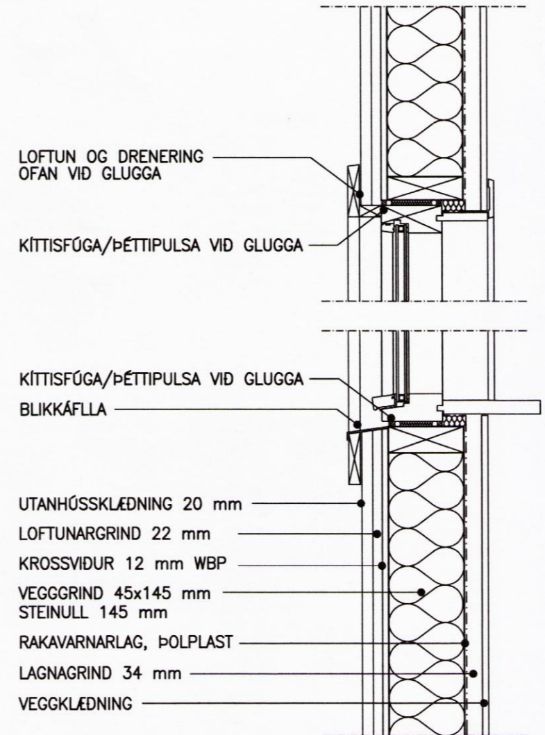
FRÁGANGUR VID GLUGGA LÓÐRÉTT SNIÐ 1:10
