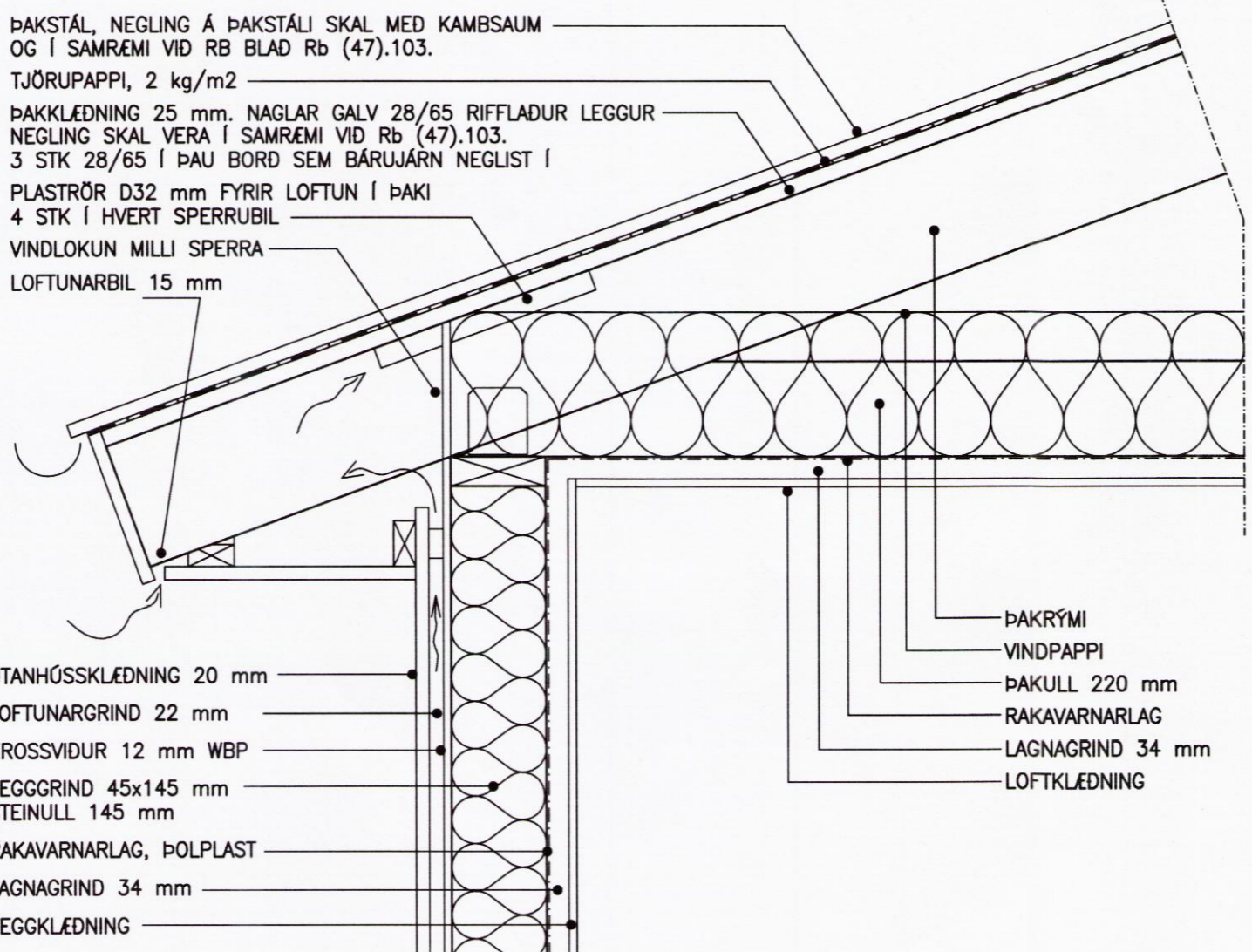
FRÁGANGUR VID ÚTVEGG OG ÞAK 1:10
