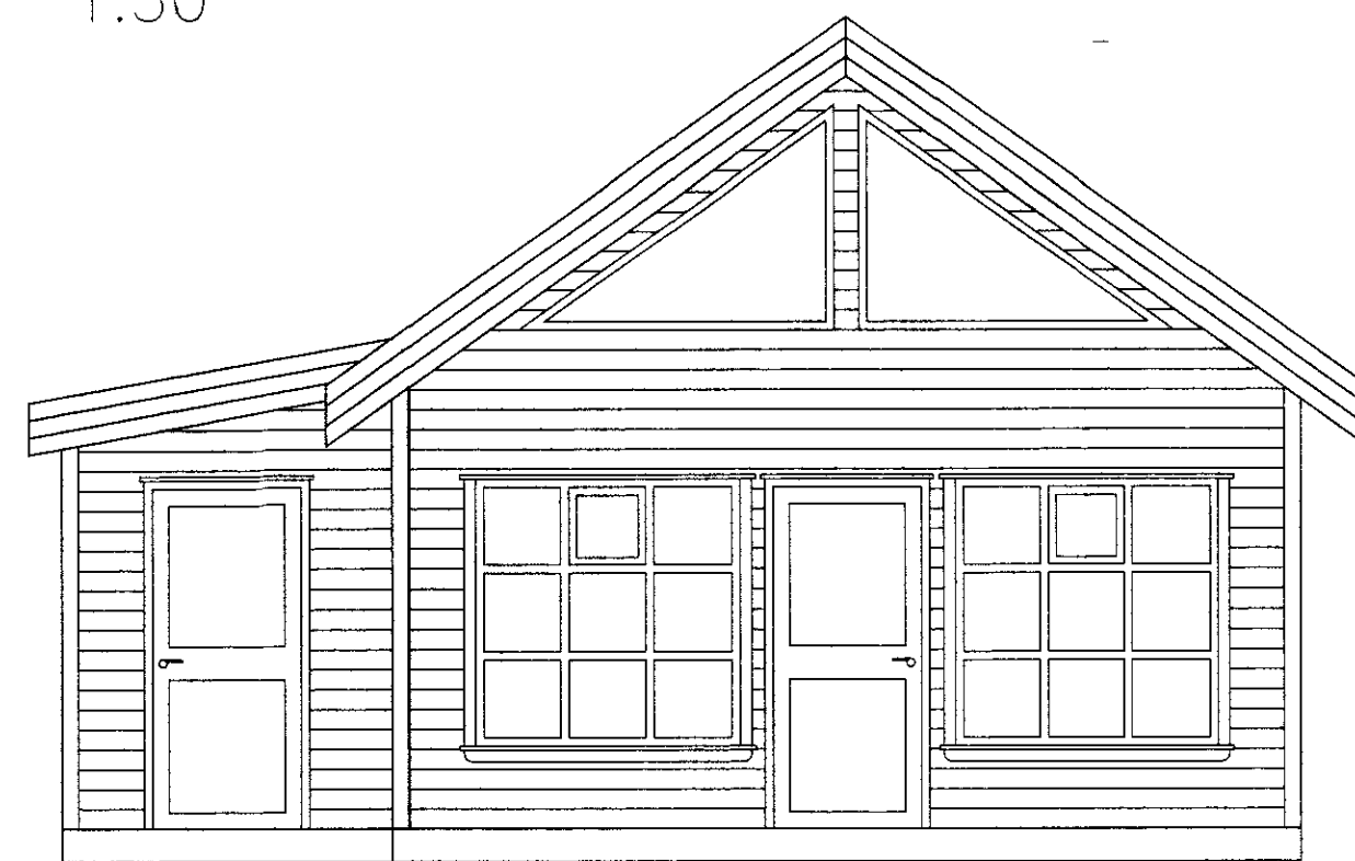
Suður 1:50
