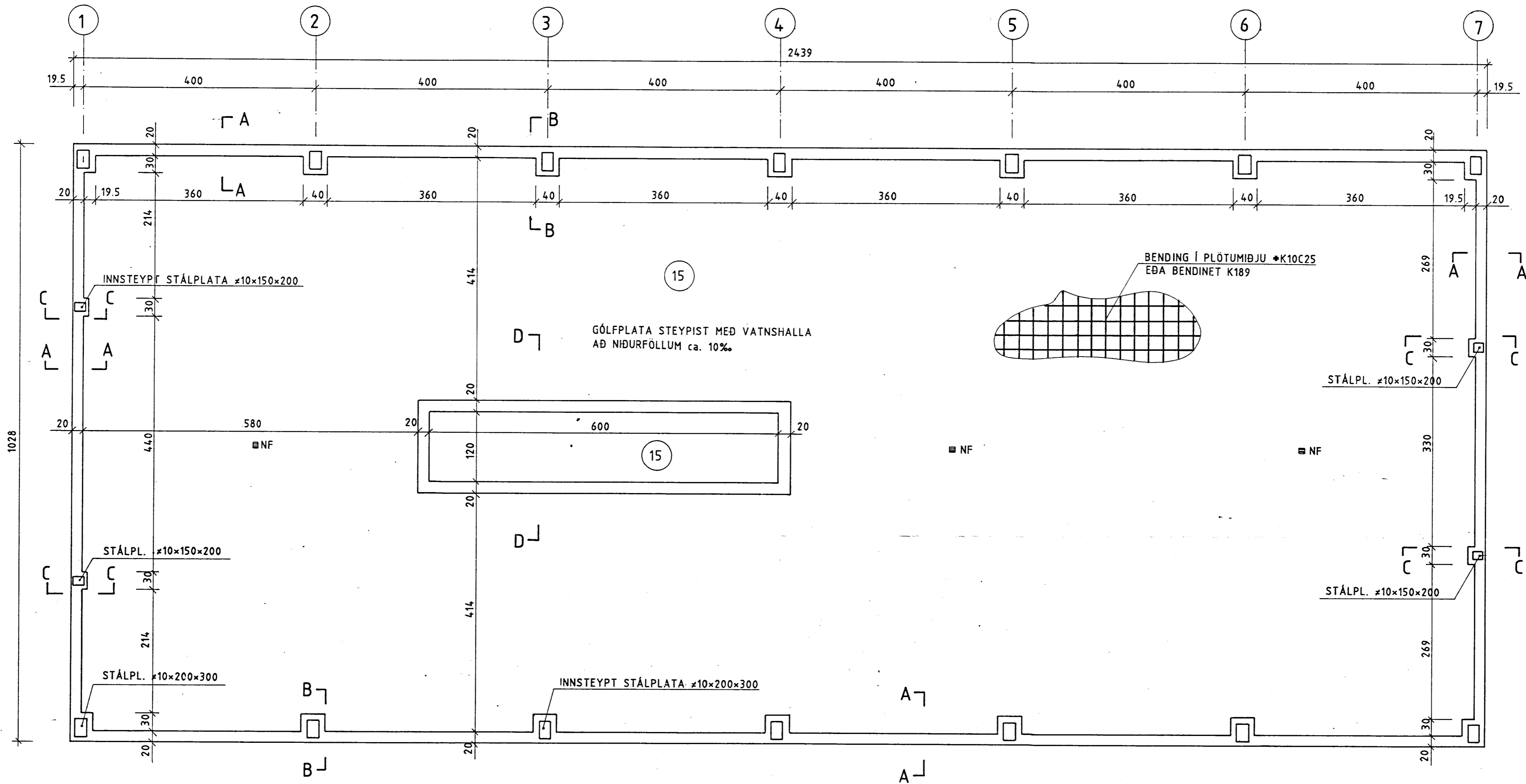
GRUNNMYND 1:50
