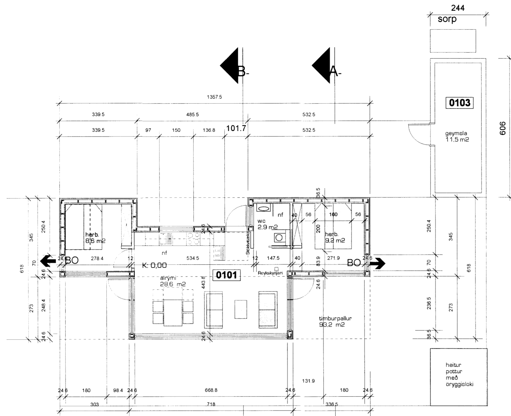
Grunnmynd mkv.:1:100
