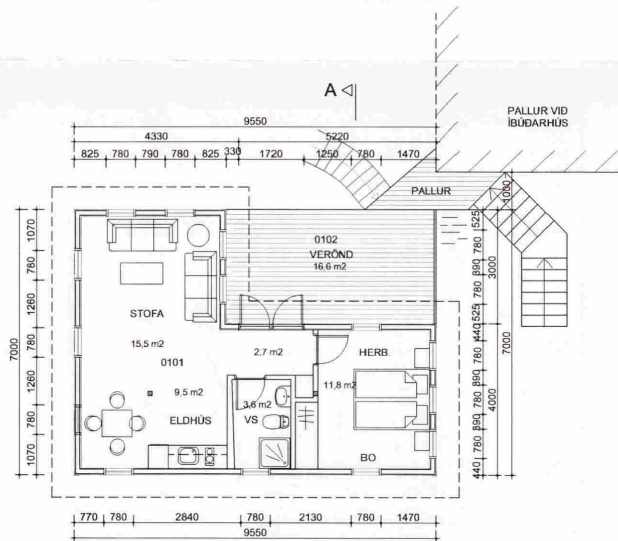
GRUNNMYND HÆÐAR
