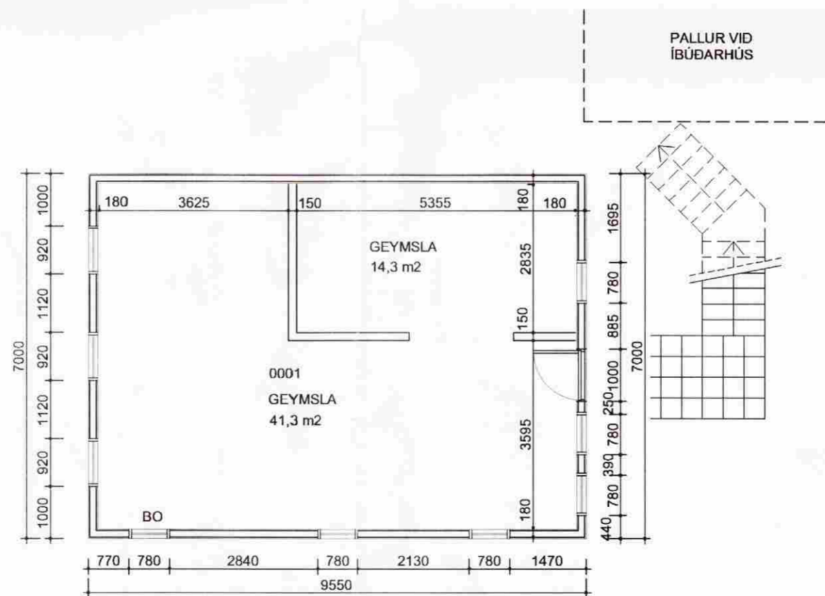
GRUNNMYND GEYMSLUKJALLARA
