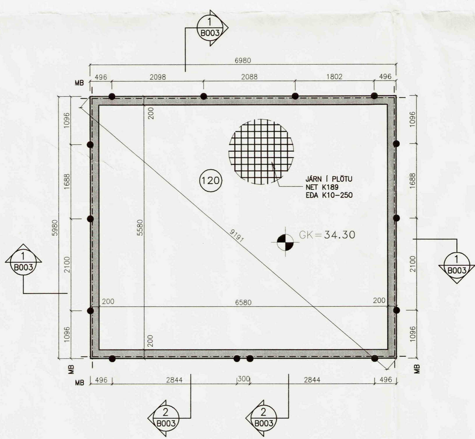
UNDIRSTÖÐUR BILGEYMSLA 1:50
