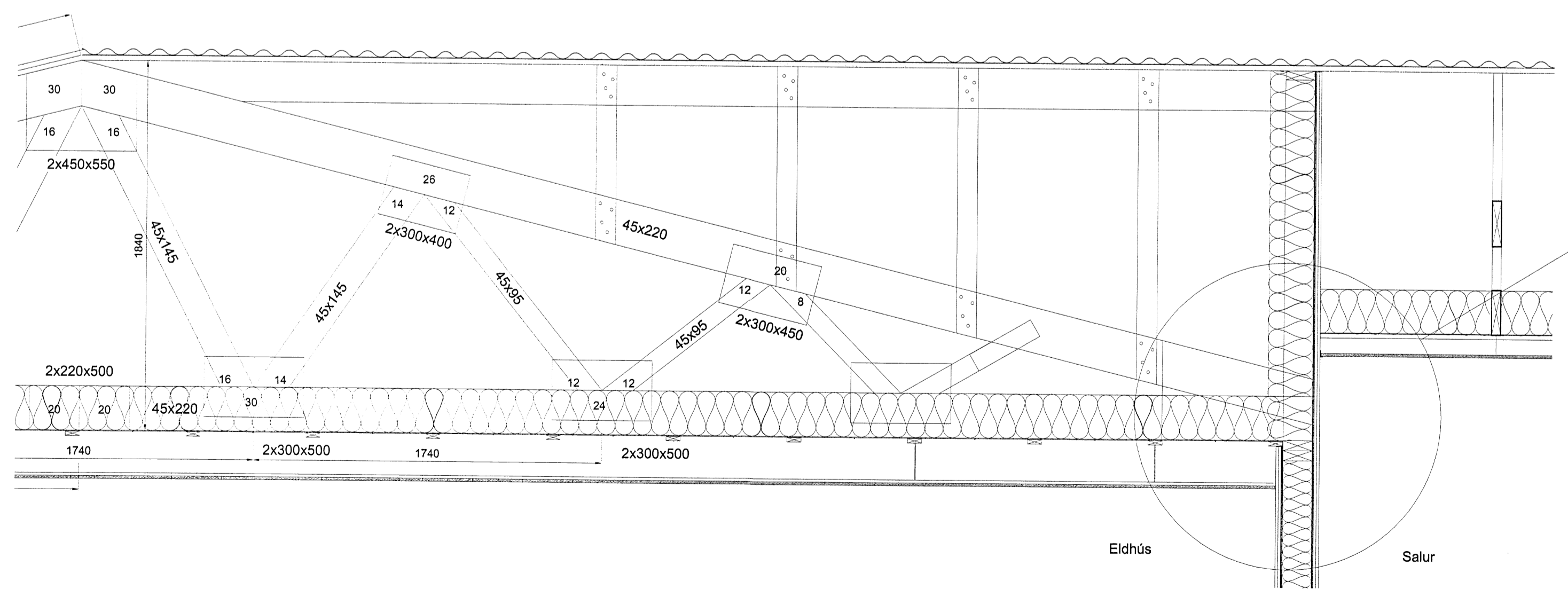
B 31-04 Frágangur á brunahólfandi veggjum Lóðréttur sérhliuti 1:20
