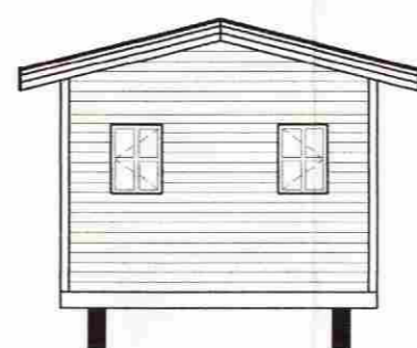
NORD-AUSTURHLID GESTAÐÚS 1:100
