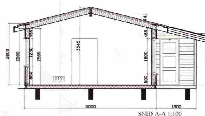
SNID A-A 1:100
