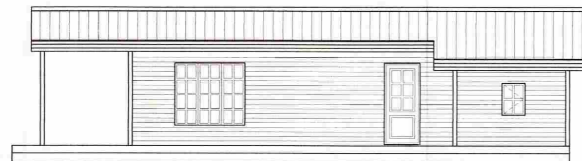
NORDVESTURHLID 1:100
