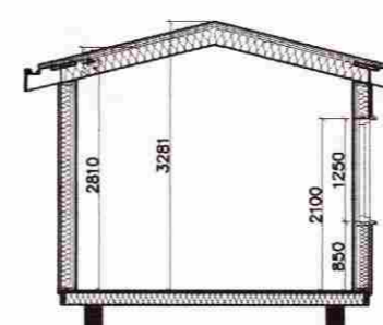
SNID B-B 1:100
