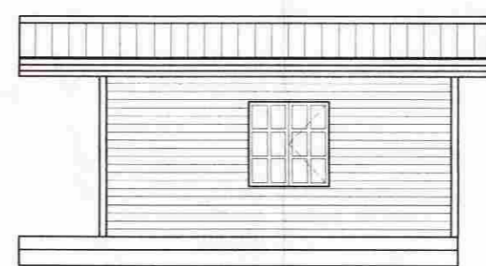
SUD-AUSTURHLID GESTAÐÚS 1:100
