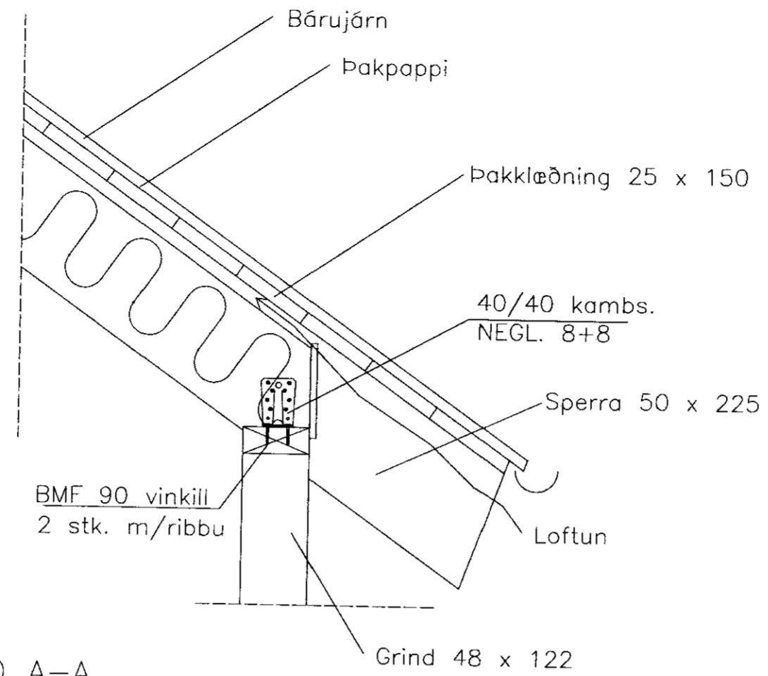
SNID A-A 1:10
