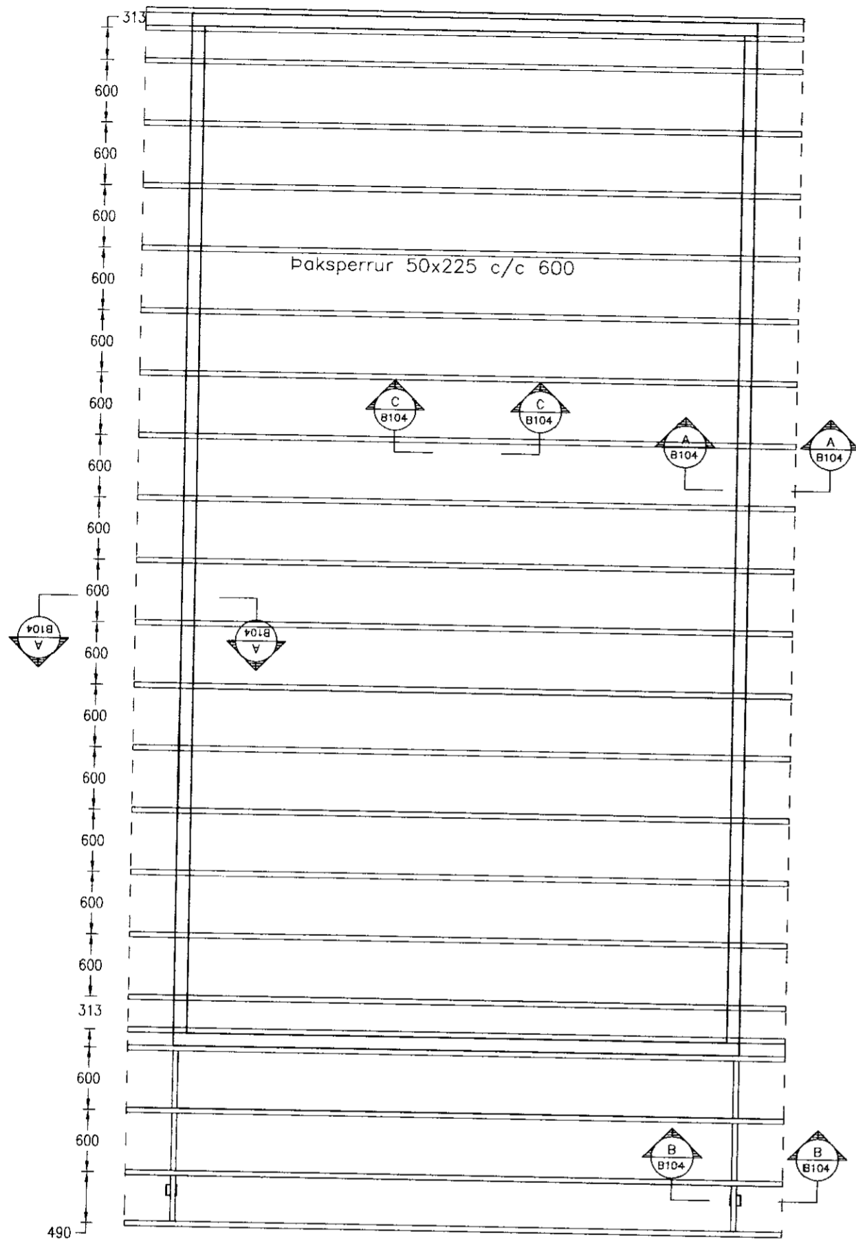
Grunnmynd 1:50
