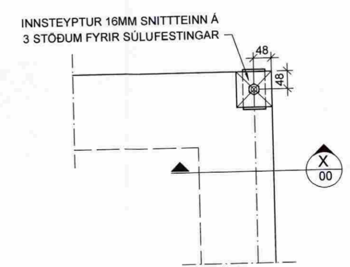
D1 DEILI 03 Mkv. 1/20
