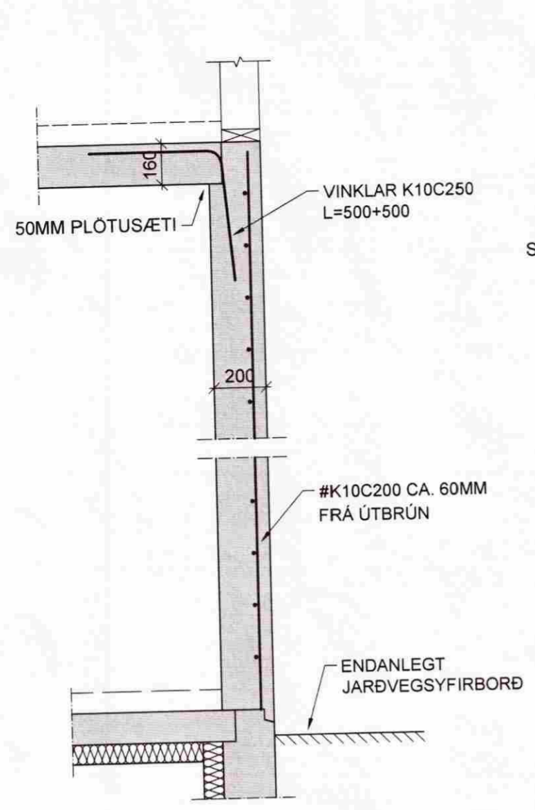
E SNEIÐING 03 Mkv. 1/20
