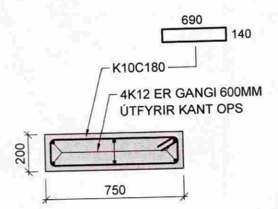
S2 SÚLA 03 Mkv. 1/20
