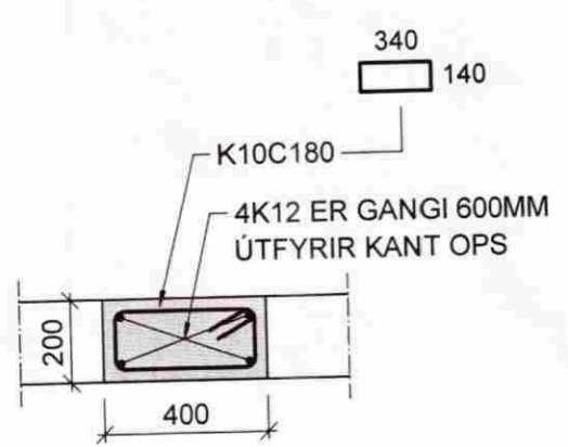
S1 SÚLA 03 Mkv. 1/20
