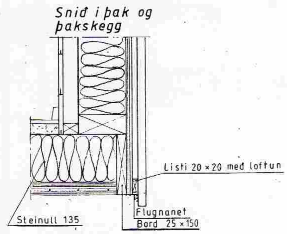
Snið þar sem veggur og gólf mætast.
