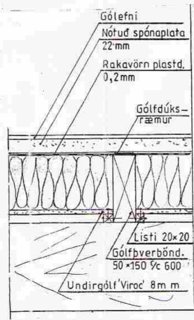
Snið í gólf
