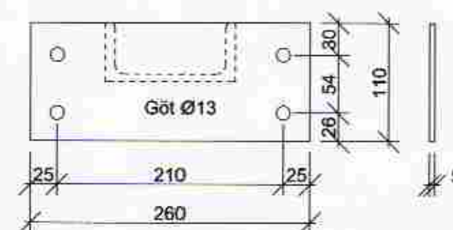
PL 260x110x5 M 1:5
