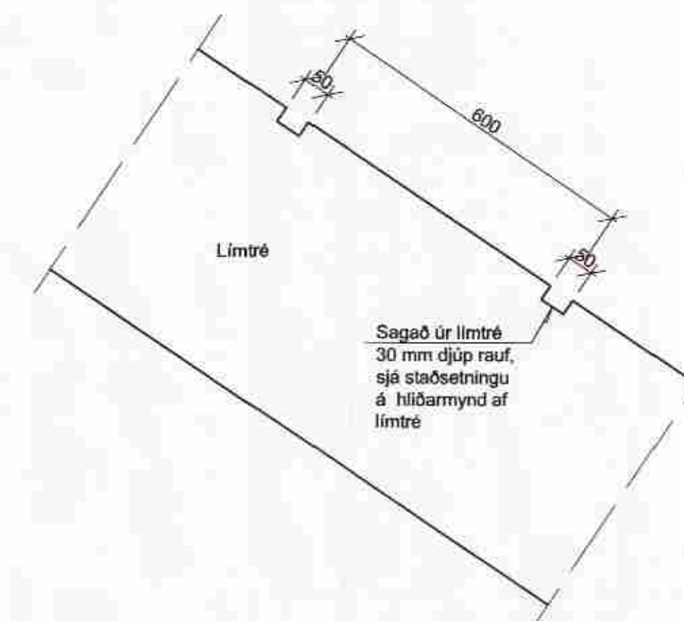
FE Snið 53 54 M 1:10
