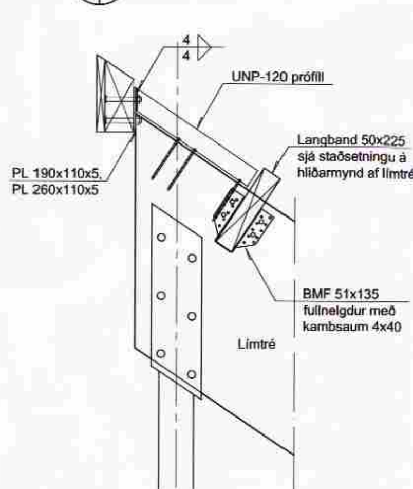
FM Snið 54 54 M 1:10
