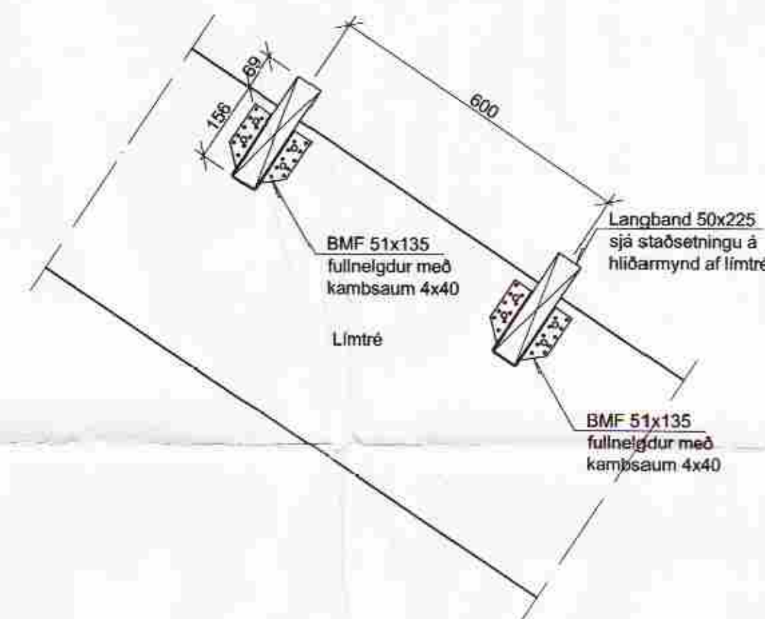
FG Snið 53 54 M 1:10
