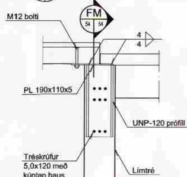
FL Mynd 53 54 M 1:10
