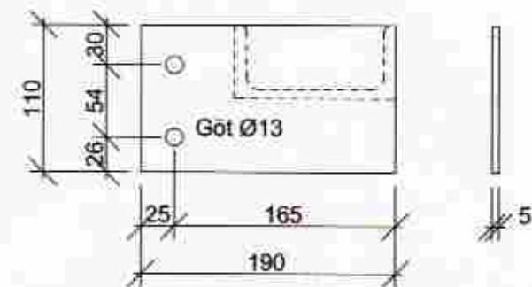
PL 190x110x5 M 1:5
