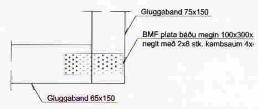
FQ Snið 54 54 M 1:10
