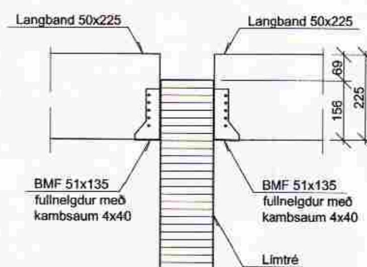
FD Snið 53 54 M 1:10
