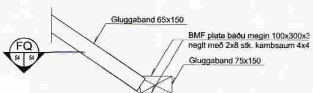
FQ Snið 54 54 M 1:10
