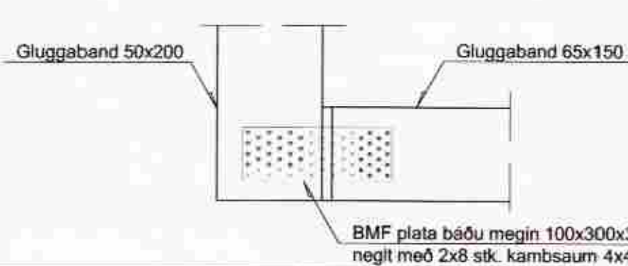
FP Snið 54 54 M 1:10
