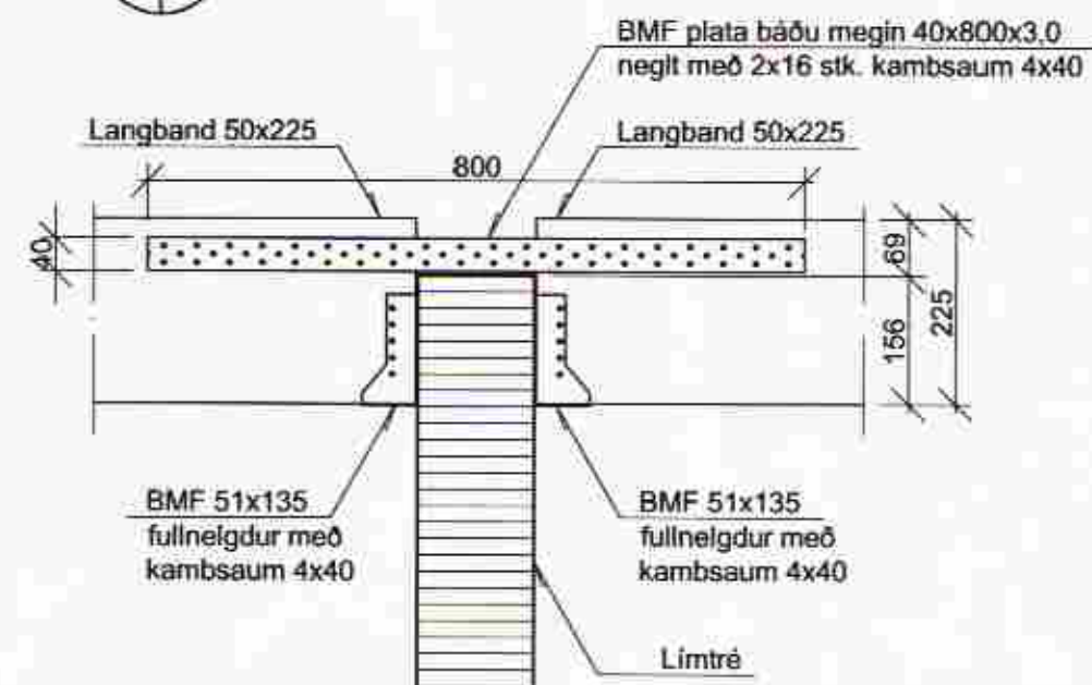
FC Snið 53 54 M 1:10
