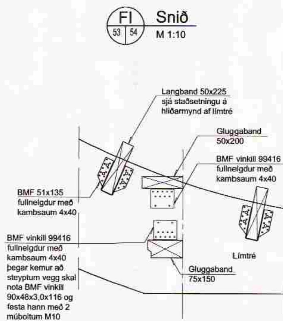
FL Mynd 53 54 M 1:10
