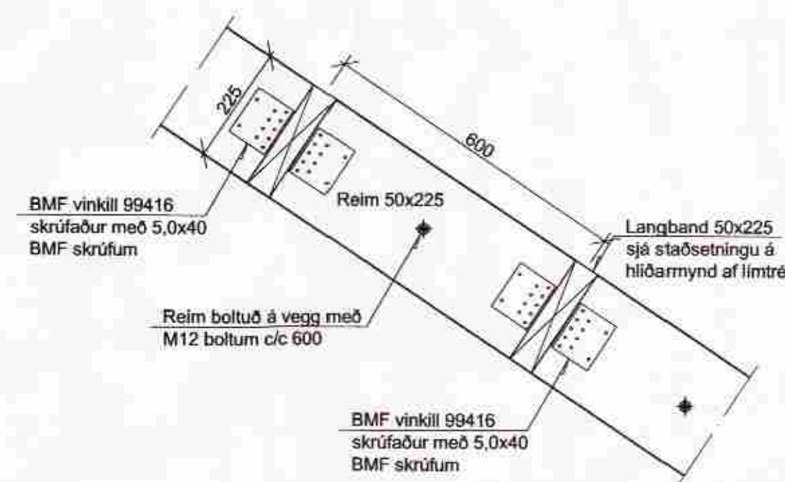
FG Snið 53 54 M 1:10
