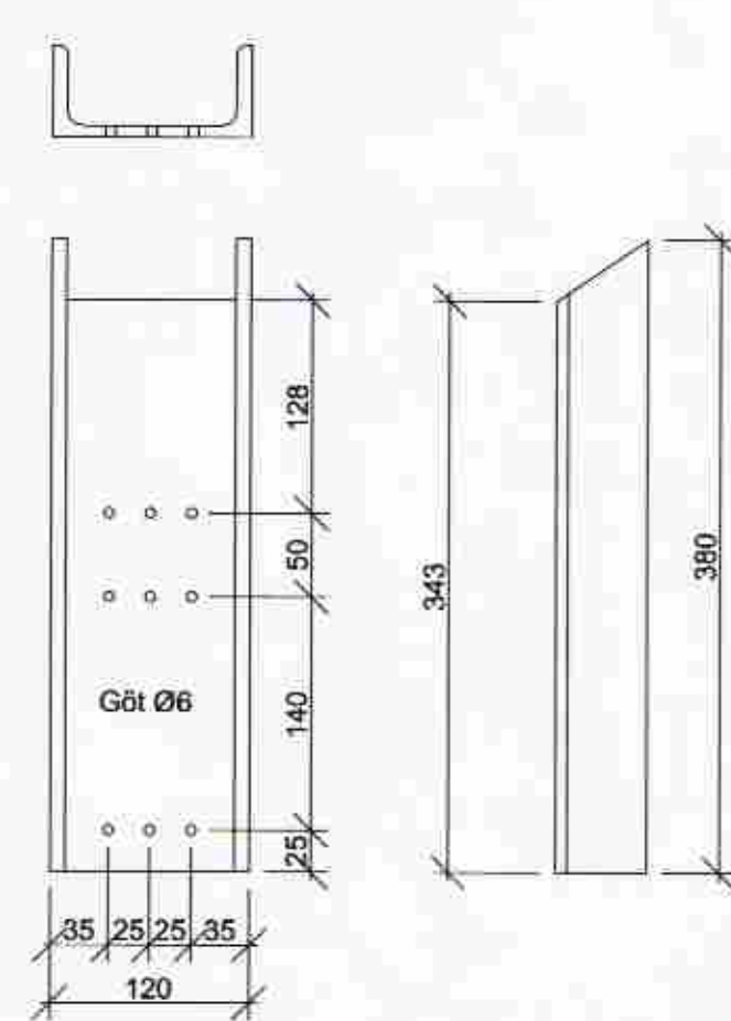
UNP-120 prófill M 1:5
