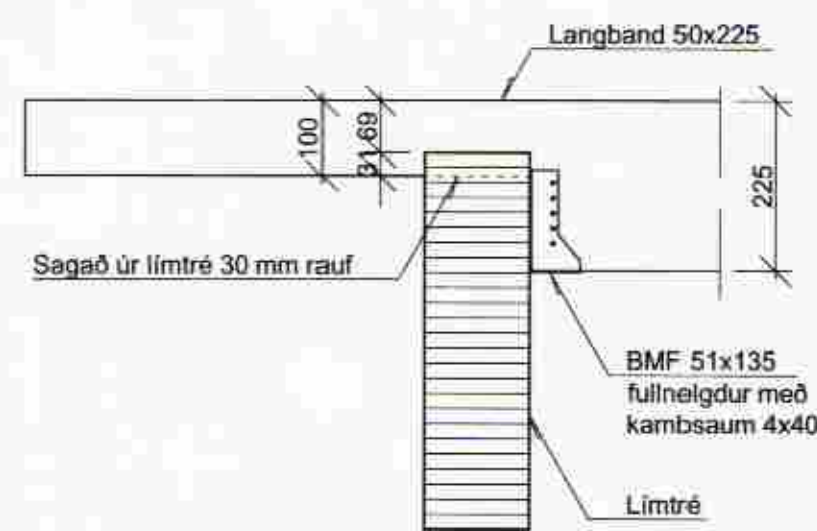
FB Snið 53 54 M 1:10
