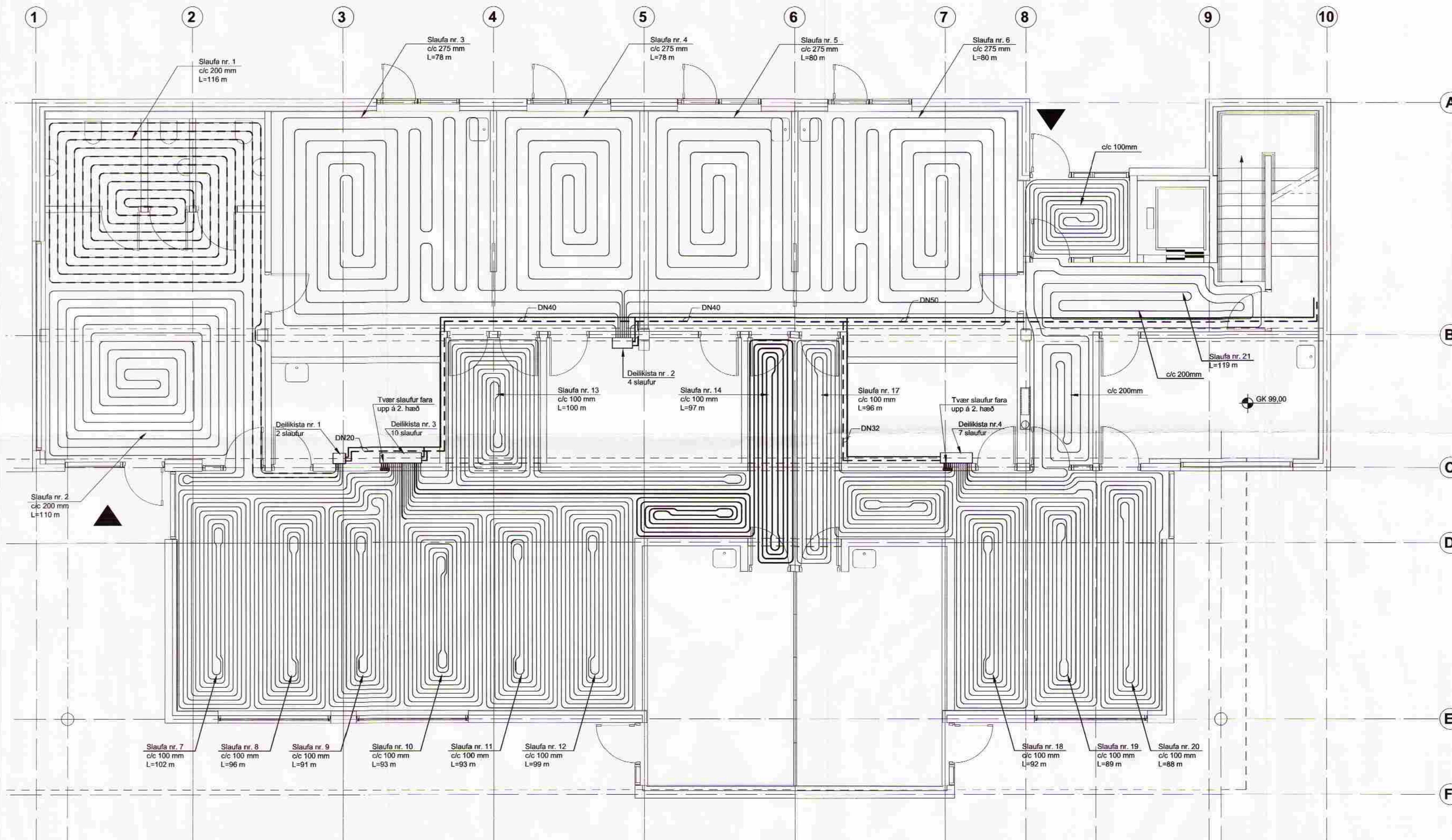
Frágangur á gólfhitalögnum í steyptri gólfplötu 1. hæðar M 1:10
