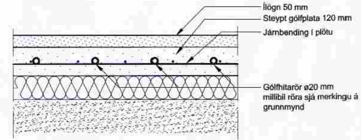
Frágangur á gólfhitalögnum í steyptri gólfplötu 1. hæðar M 1:10
