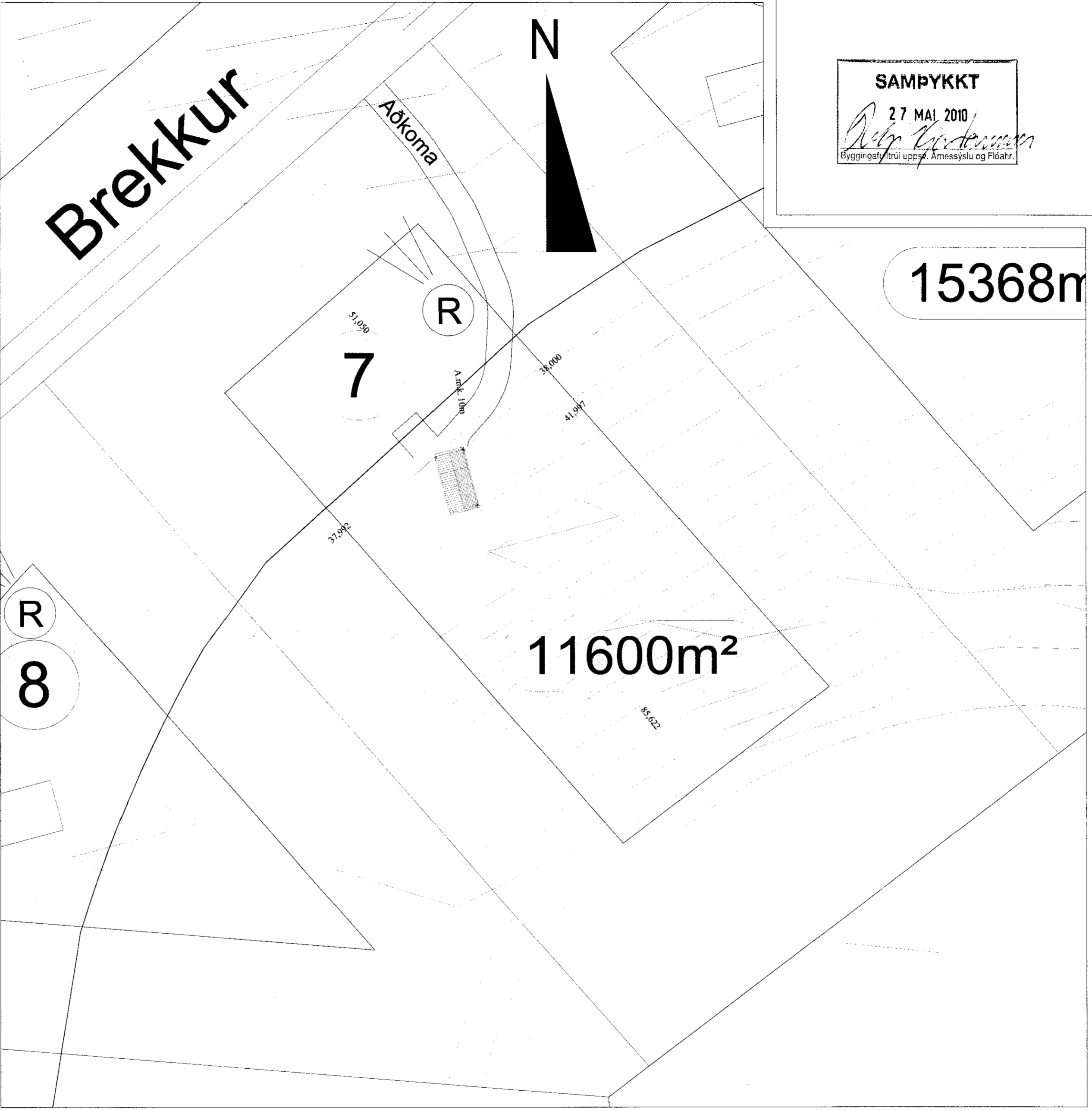
Afstöðumynd mkv. 1:500
