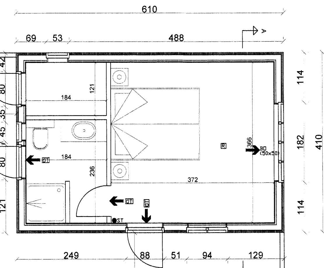
GRUNNMYND GESTAHÚS
