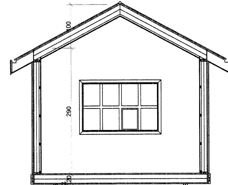
SNIÐ A-A
