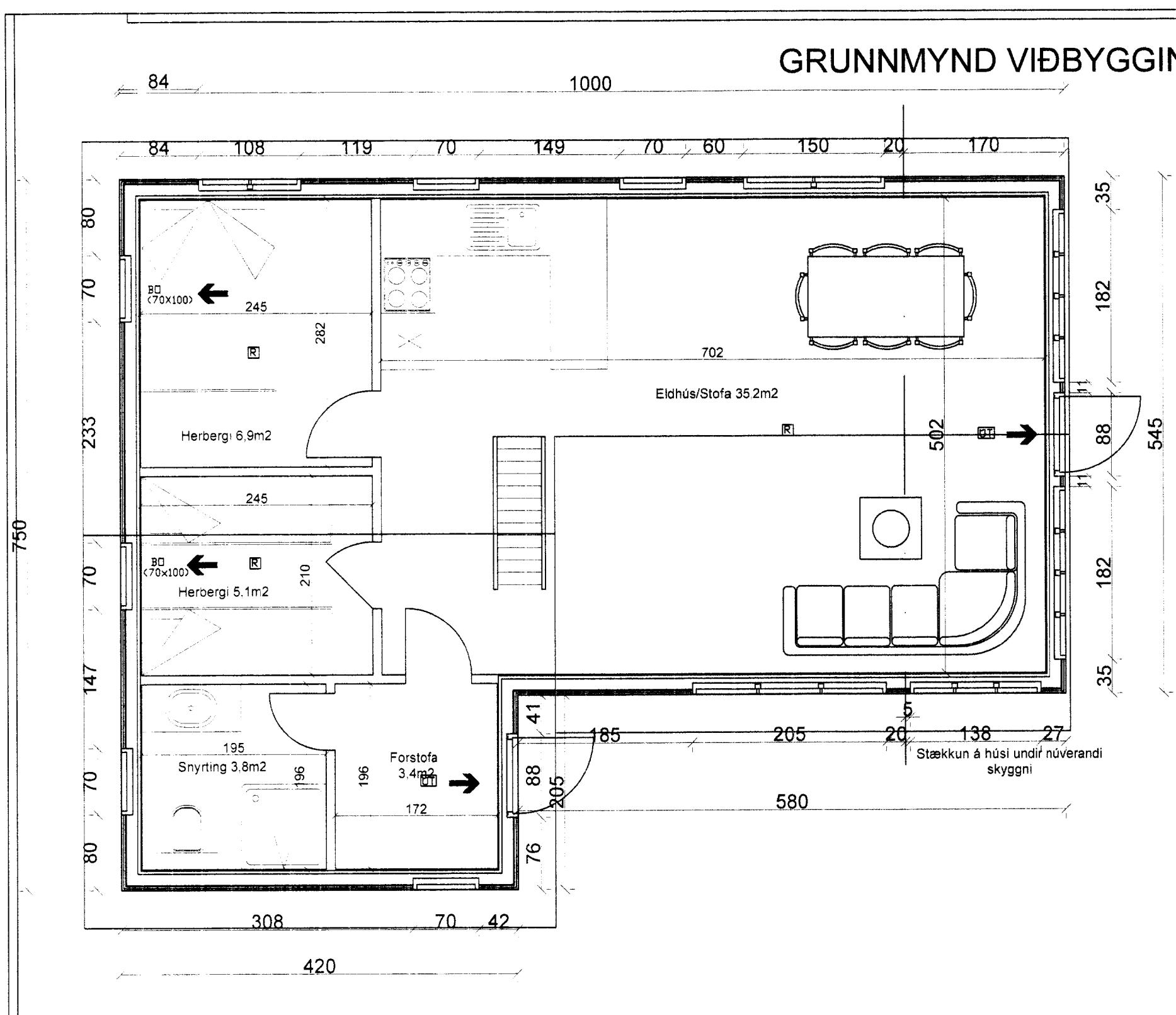
GRUNNMYND NÚVERANDI HÚS
