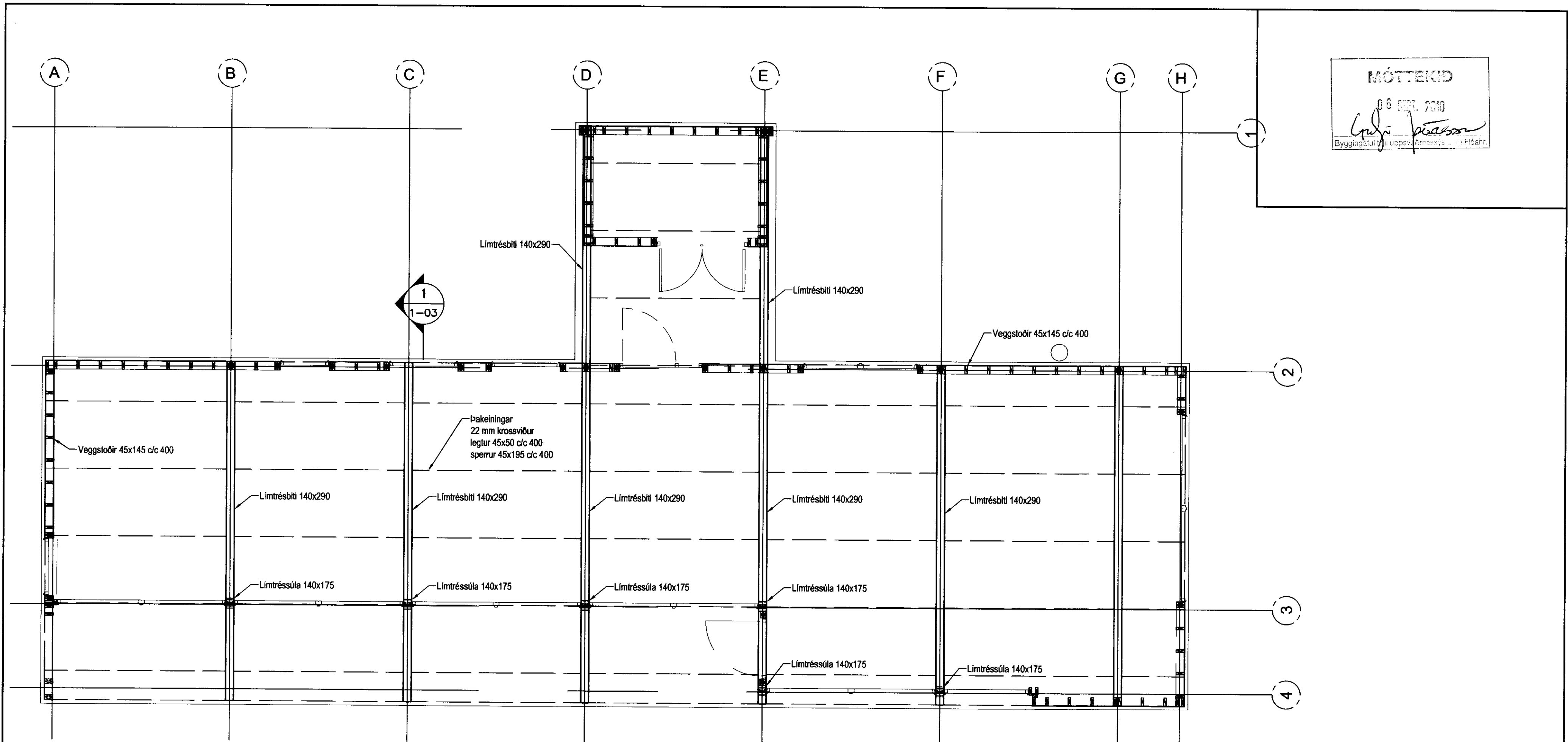
Grunnmynd, 1:50
