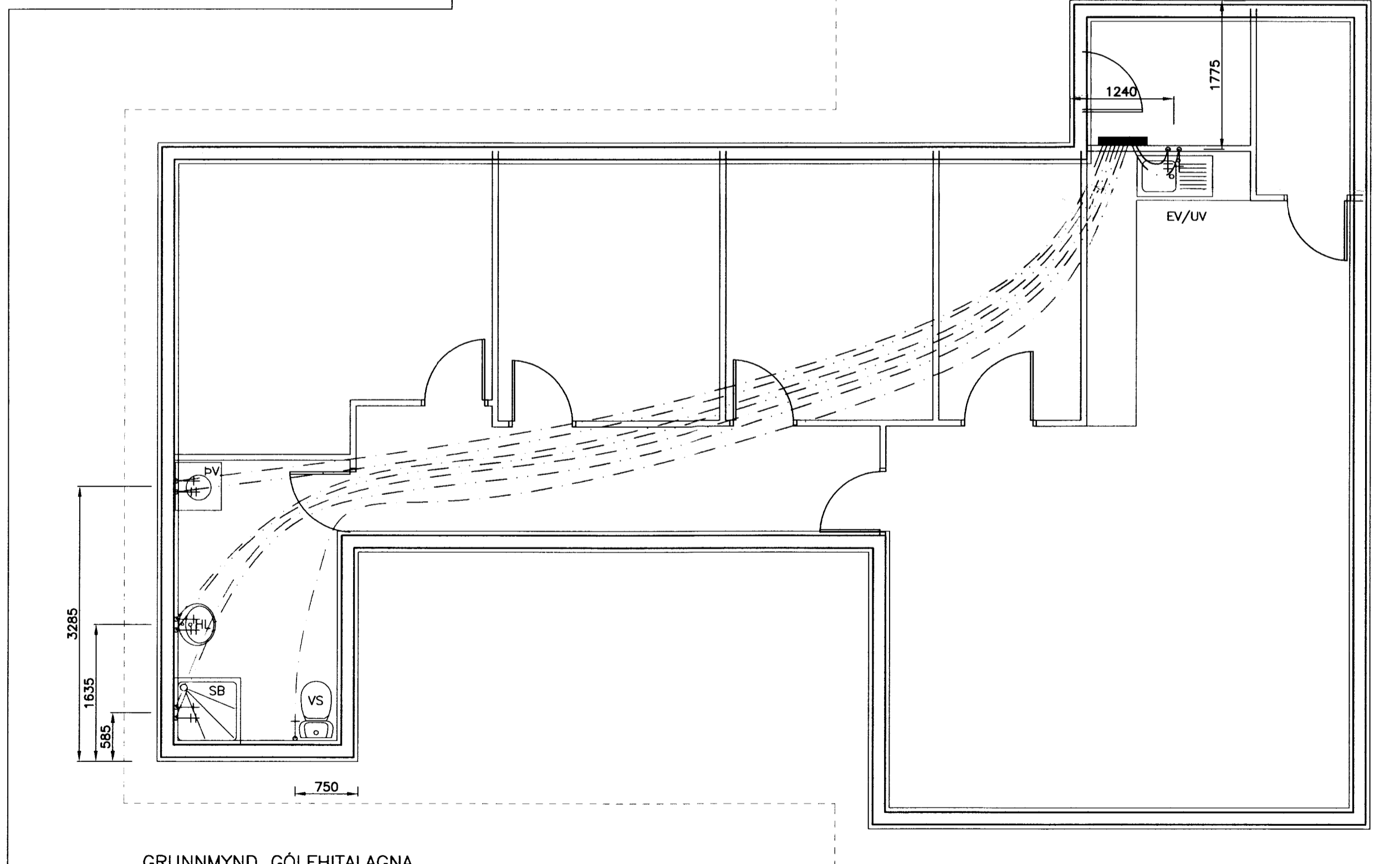
GRUNNMYND GÓLFHITALAGNA MKV. 1:50
