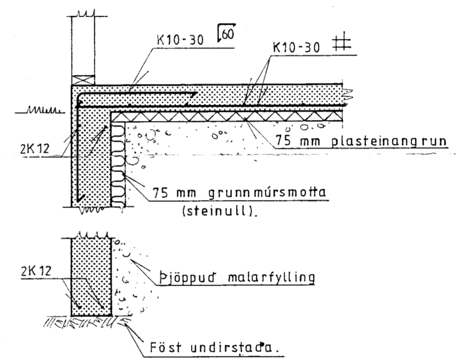
Snid í sökklá M = 1:20
